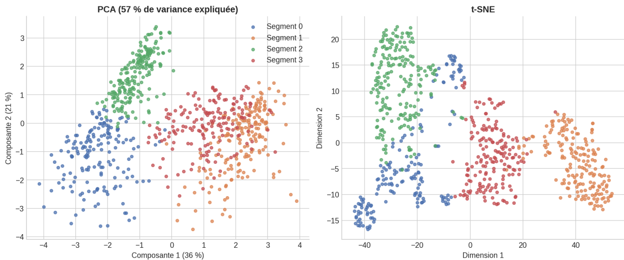
Figure 7 — Projection des segments par PCA et t-SNE.
