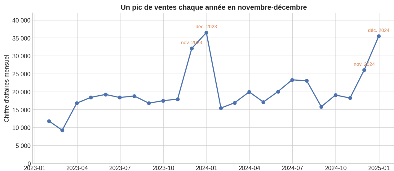
Figure 4 — Évolution mensuelle du chiffre d'affaires.
