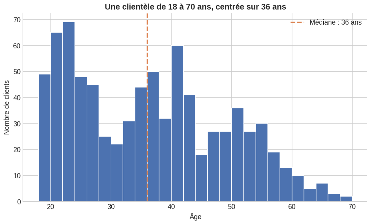
Figure 1 — Distribution de l'âge des clients.
