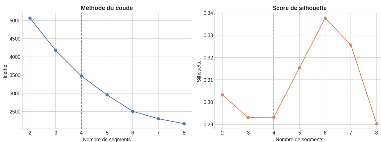
Figure 6 — Méthode du coude et score de silhouette.
