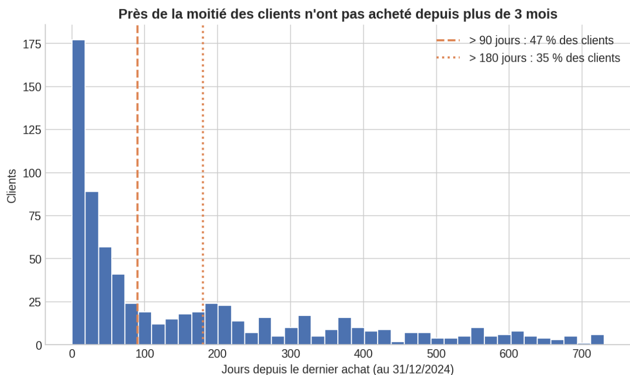
Figure 5 — Jours écoulés depuis le dernier achat.
