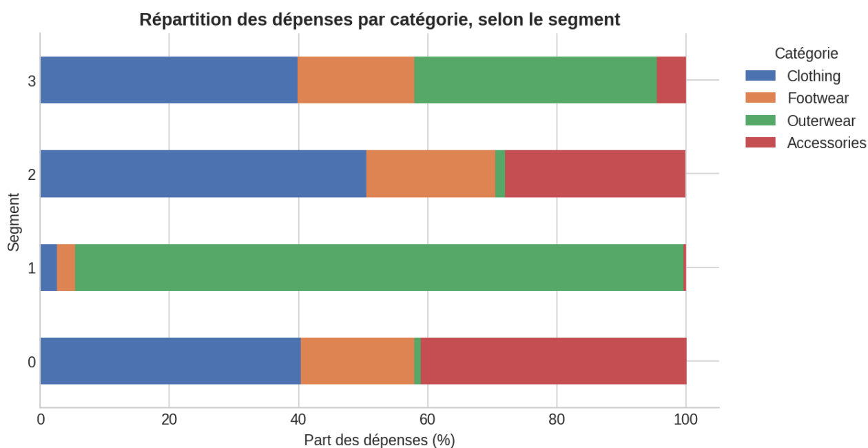
Figure 8 — Répartition des dépenses par catégorie, selon le segment.
