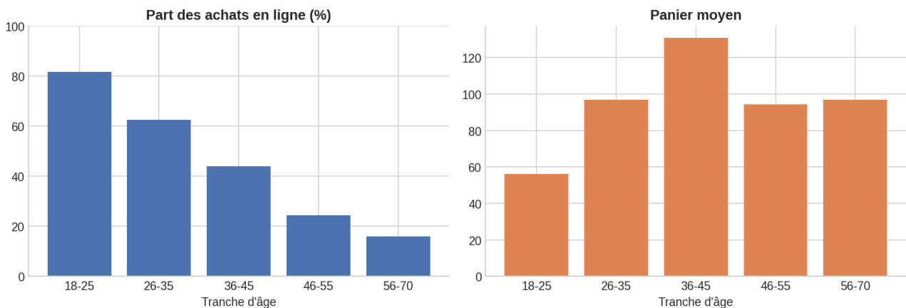
Figure 3 — Part des achats en ligne et panier moyen par tranche d'âge.
