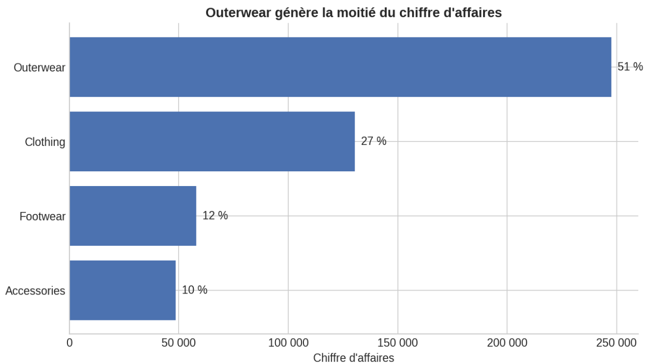
Figure 2 — Chiffre d'affaires par catégorie de produits.
