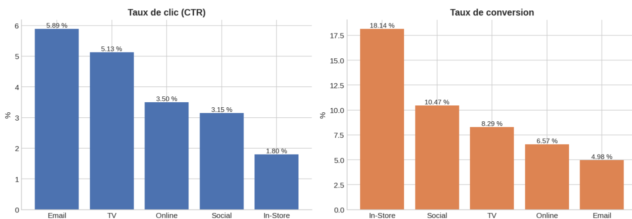
Figure 9 — Taux de clic et taux de conversion par canal.
