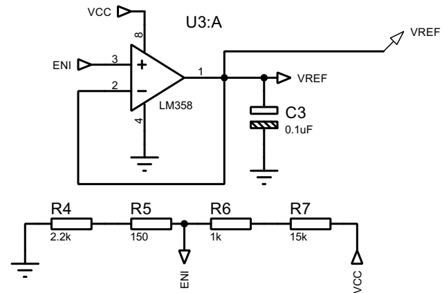
MODULO_SEGUIDOR_VREF
