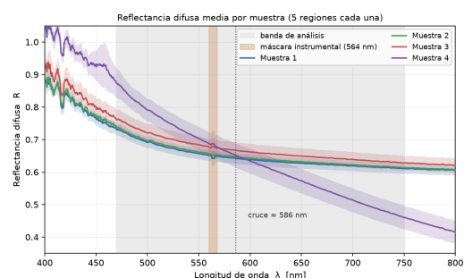
FIGURA 1. Reflectancia media por muestra. Gris: banda de análisis. Franja naranja: zona excluida por un pico instrumental. Punteada vertical: cruce de curvas.
