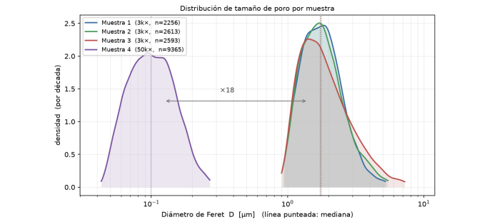
FIGURA 3. Distribución de tamaño de poro por muestra, en escala logarítmica; n es la cantidad de poros medidos y las punteadas marcan las medianas.
