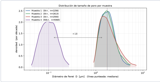
Figura 3. Distribución de tamaño de poro por muestra, en escala logarítmica; n es la cantidad de poros medidos y las punteadas marcan las medianas.
