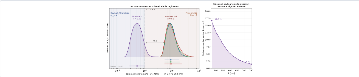
Figura 4. Izquierda: distribución de x por muestra; las barras inferiores contienen al 90 % de los poros y la punteada marca x = 1 . Derecha: fracción de poros de la muestra 4 que supera esa frontera según la longitud de onda.
