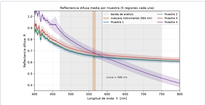
Figura 1. Reflectancia media por muestra. Gris: banda de análisis. Franja naranja: zona excluida por un pico instrumental. Punteada vertical: cruce de curvas.
