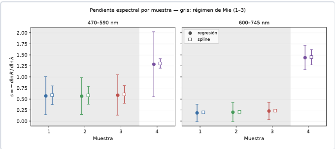
Figura 2. Pendiente por muestra. Círculos: regresión log-log. Cuadrados: derivada de un spline. Barras: incertidumbre del ajuste. Fondo gris: las micrométricas.
