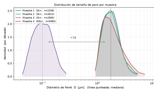
FIGURA 3. Distribución de tamaño de poro por muestra, en escala logarítmica; n es la cantidad de poros medidos y las punteadas marcan las medianas.
