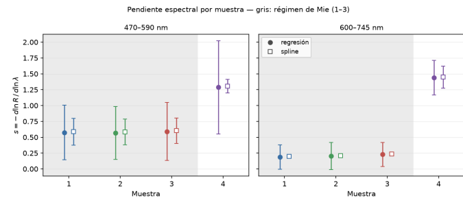
FIGURA 2. Pendiente por muestra. Círculos: regresión log-log. Cuadrados: derivada de un spline. Barras: incertidumbre del ajuste. Fondo gris: las micrométricas.
