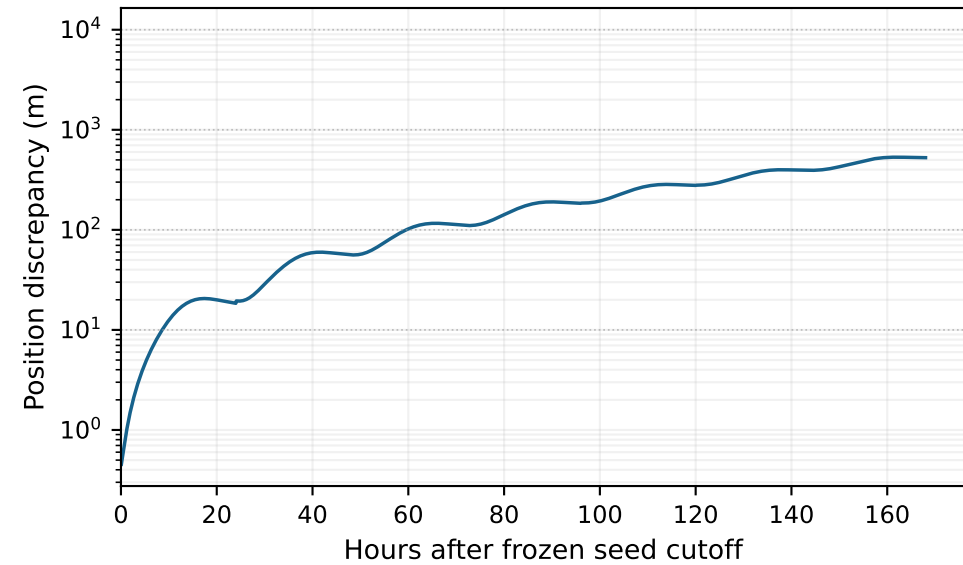
C03 / GEO
