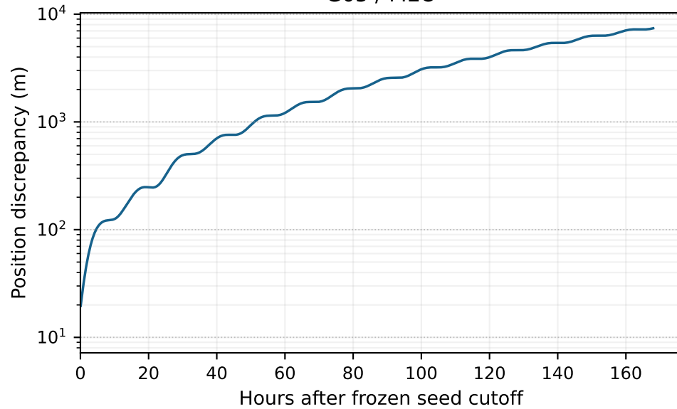
G05 / MEO
