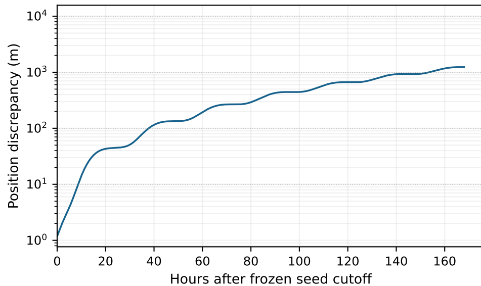
C06 / IGSO
