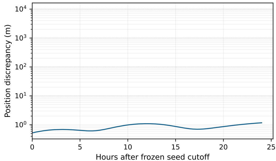
C06 / IGSO
