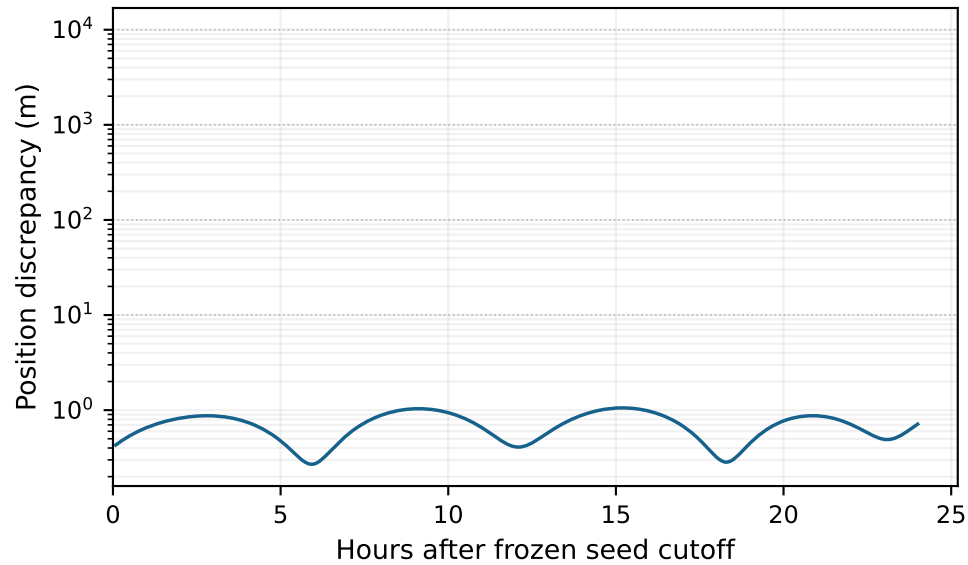
G05 / MEO
