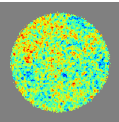
CMB - I - Output
