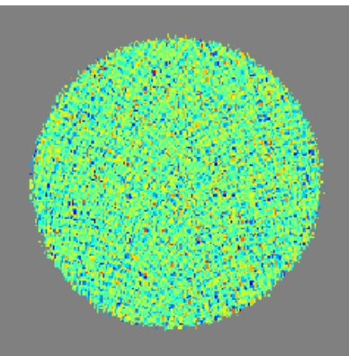
CMB - U - Output
