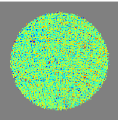
CMB - Q - Output
