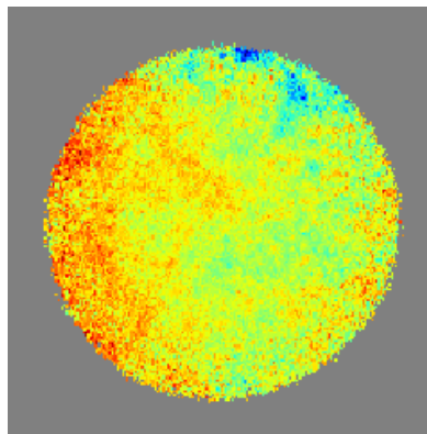
Dust - U - Output
