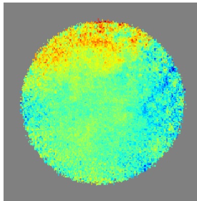
Dust - Q - Output
