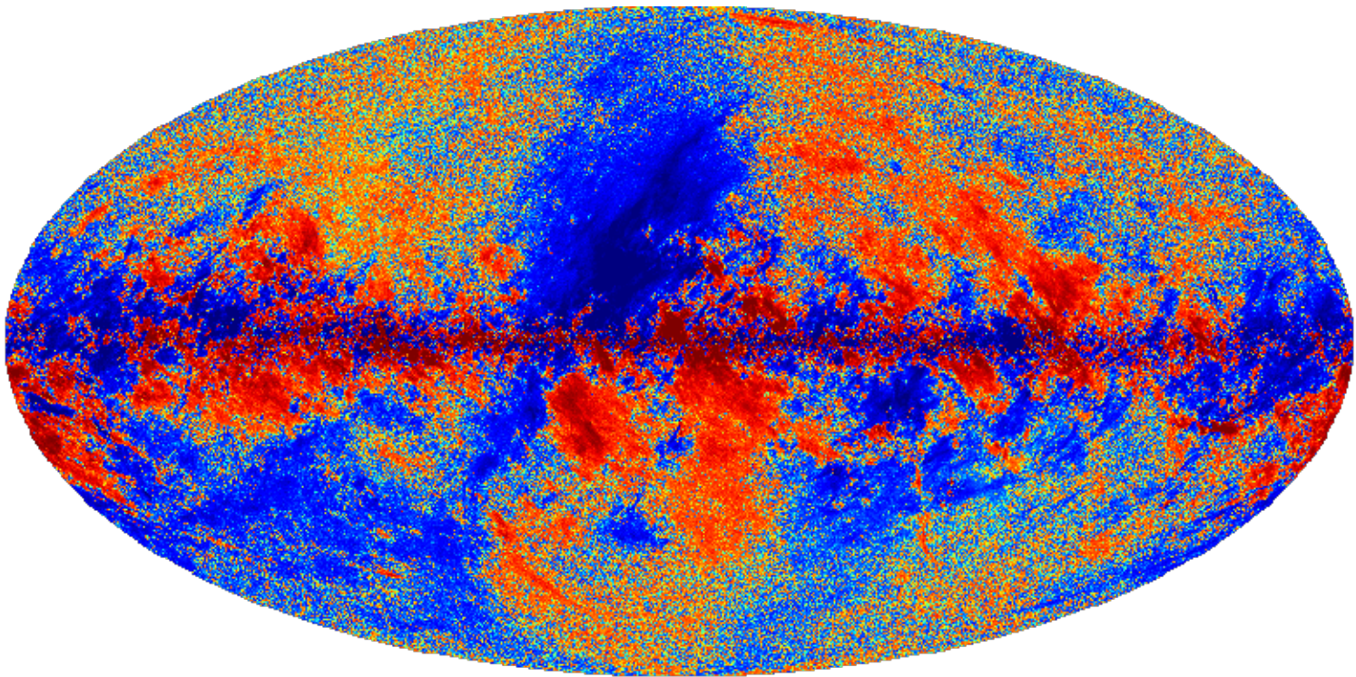
Dust U — 353 GHz
