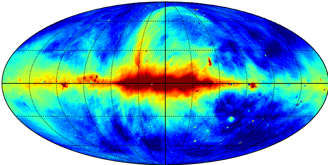
Synchrotron / — 30 GHz
