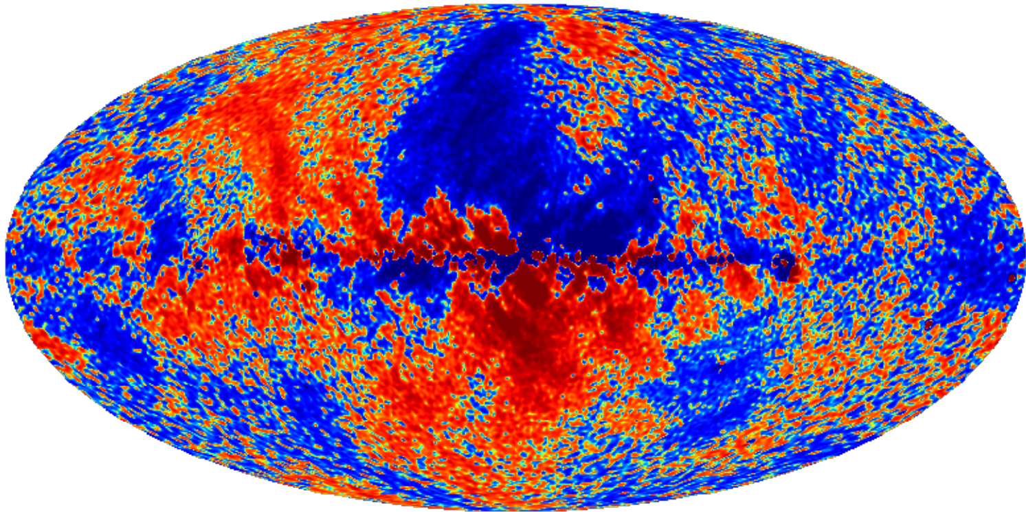
Synchrotron U — 30 GHz
