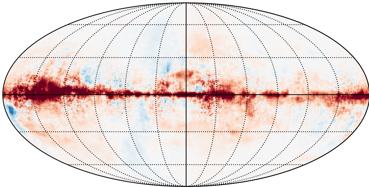
Dust Q — 353 GHz
