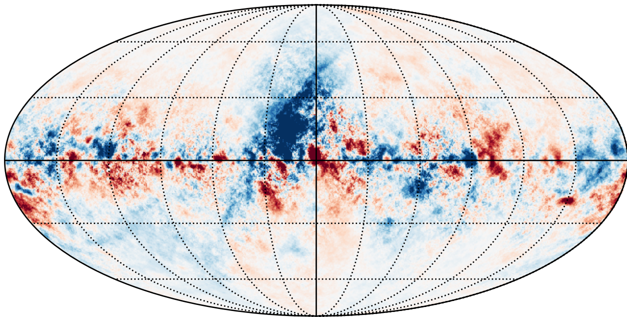
Dust U — 353 GHz
