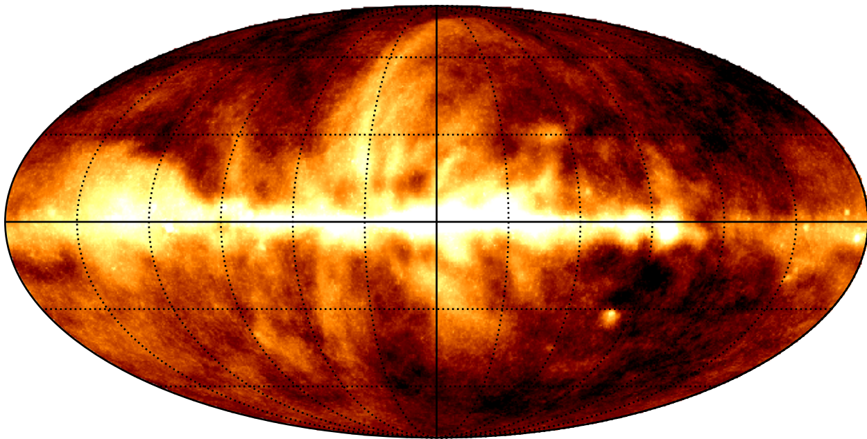
Synchrotron I — 30 GHz
