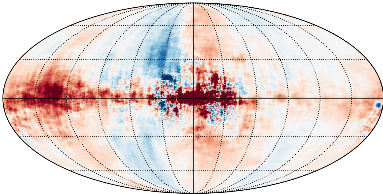
Synchrotron Q — 30 GHz
