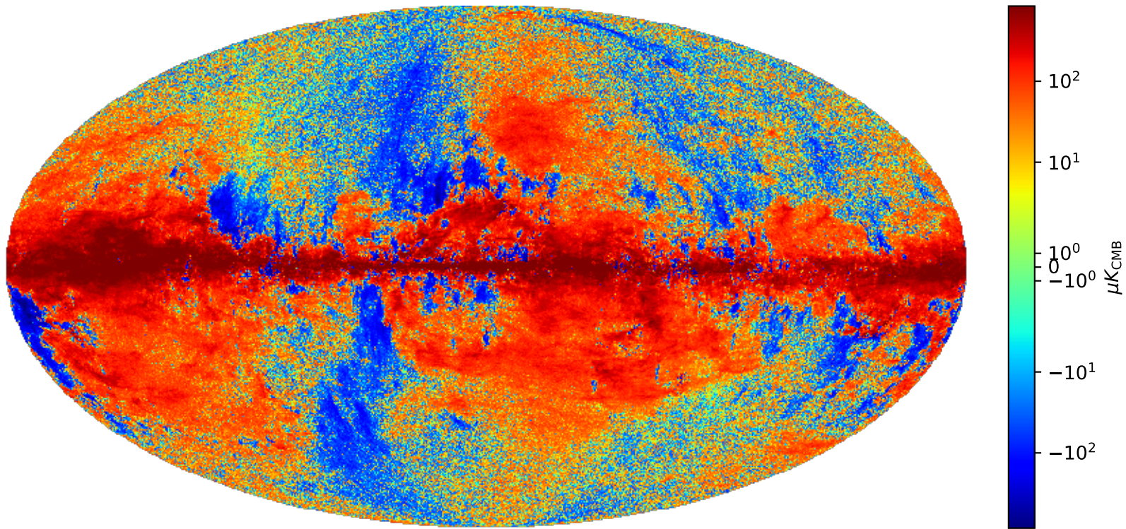
Dust Q — 353 GHz
