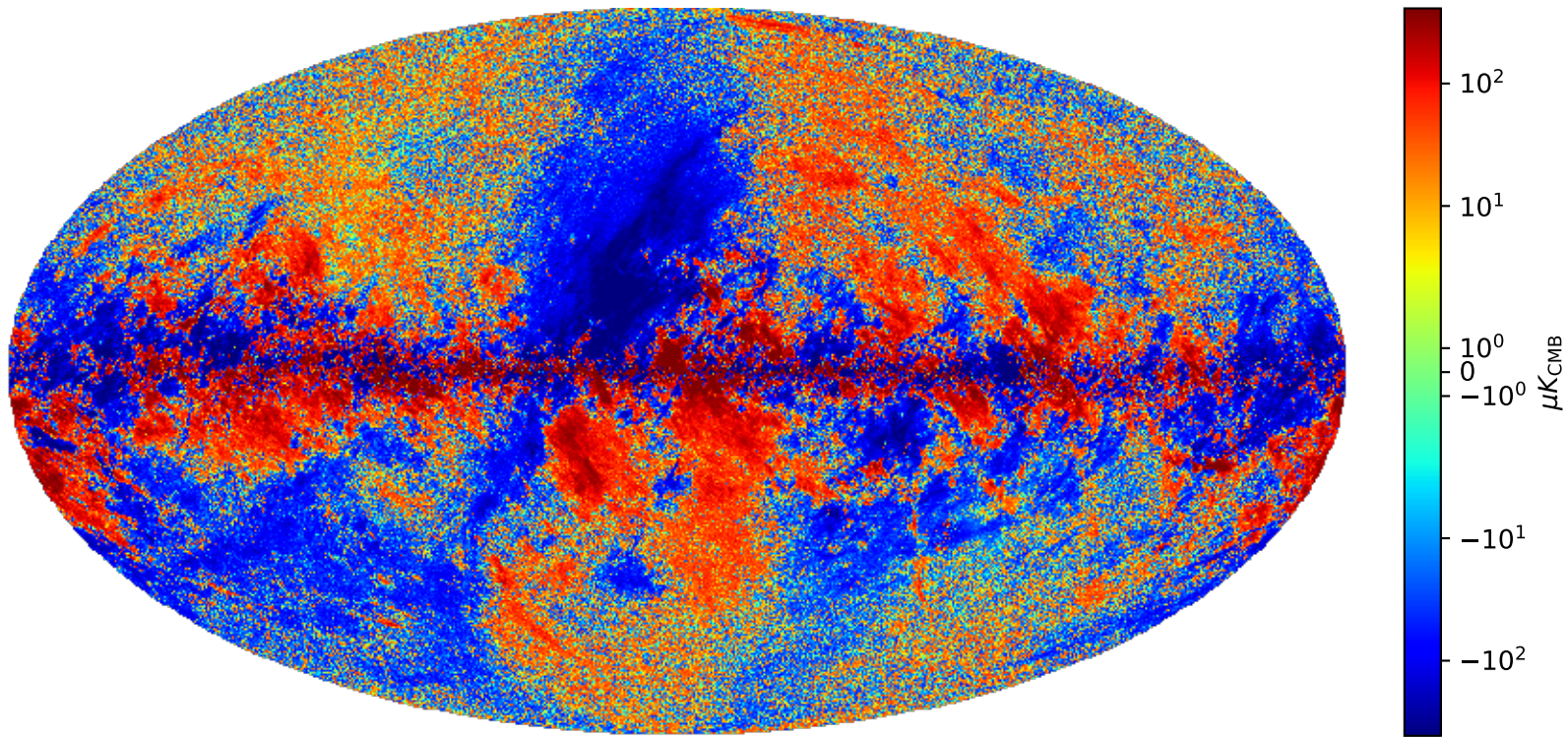
Dust U — 353 GHz
