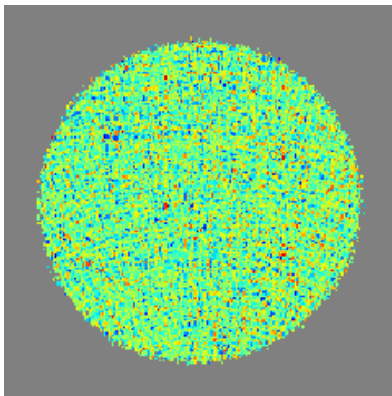
CMB - Q - Output
