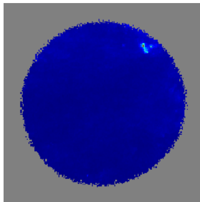
Dust - I - Output
