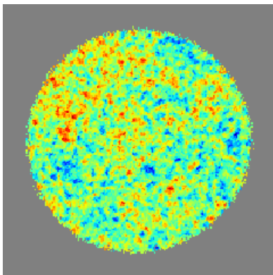
CMB - I - Output
