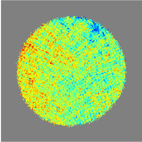
233.0 GHz - U input
