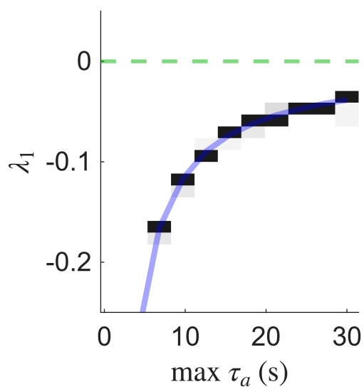
Figure 21: fig_sfa_EOC_allStd/Fig_SFA_EOC_allStd.png
