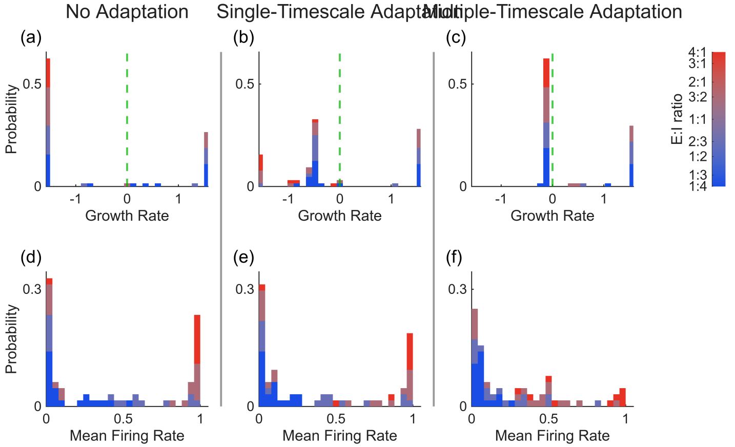
Figure 4: fig_EI_param_space/Fig_EI_ParamSpace.png
