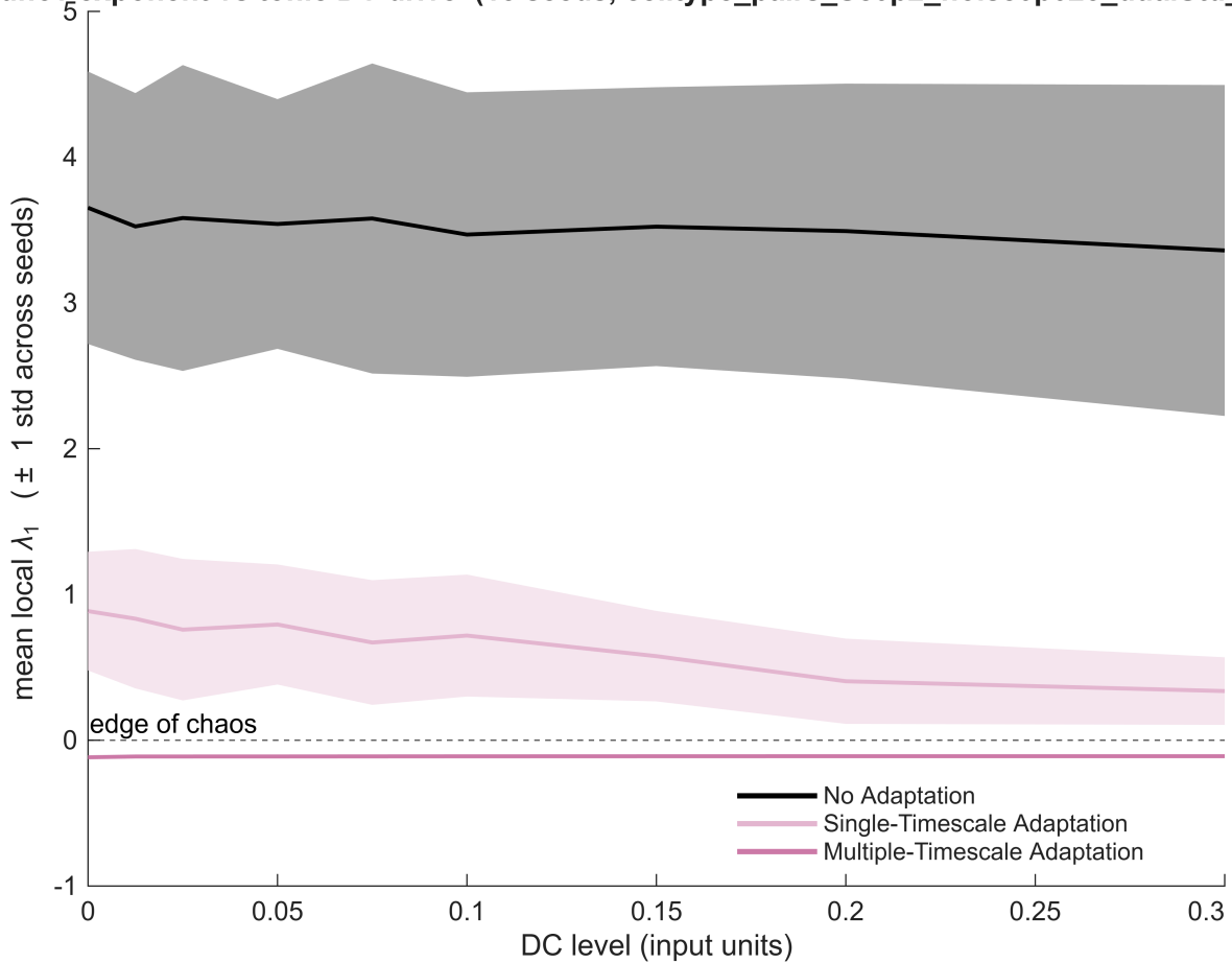
Figure 3: fig_dc_lle/fig_dc_lle.png
