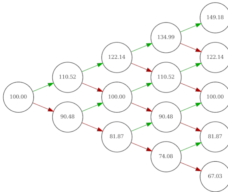
Figure 3: Propagation des prix de l'actif
