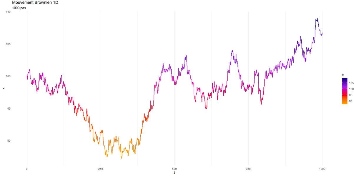
Figure 8: Simulation du mouvement brownien 1D
