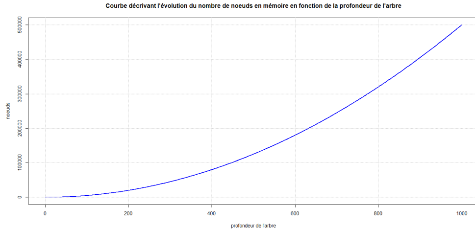
Figure 5: Evolution du nombre de nœuds en fonction de la profondeur de l'arbre
