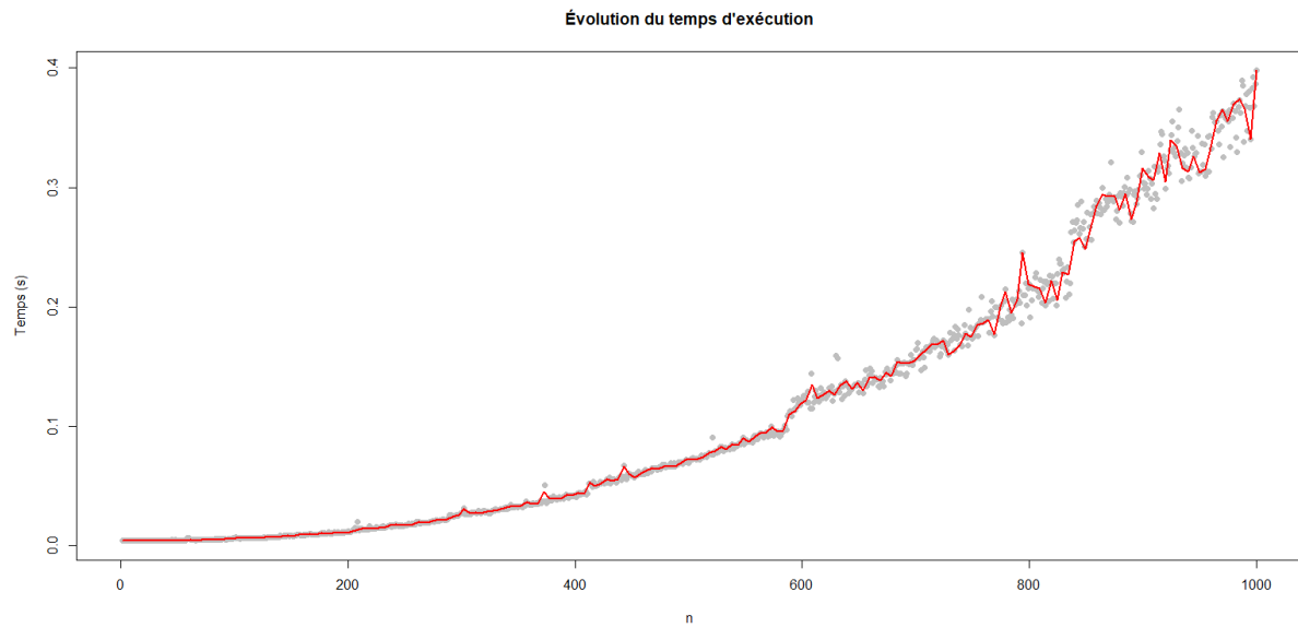
FIGURE 4 – Evolution du temps d'exécution en fonction de la profondeur de l'arbre
