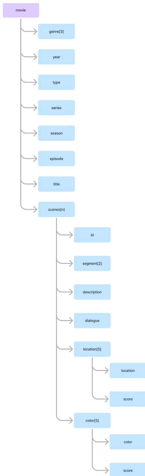
Figura 40 — Esquema representativo da organização de dados no ficheiro json
