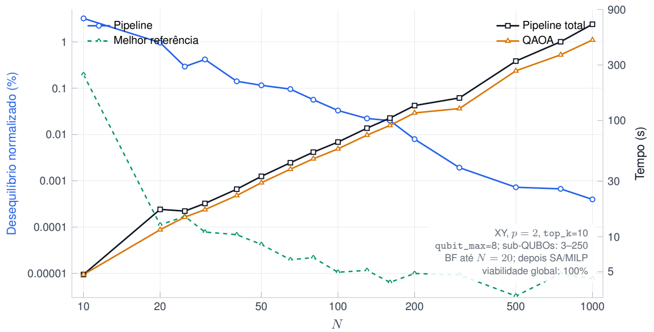
Figure 1: Escalabilidade corrigida da pipeline iterativa na Fase 5. O eixo esquerdo compara o desequilíbrio normalizado médio da pipeline com a melhor referência disponível: brute force nas instâncias pequenas e simulated annealing ou testemunho MILP nas restantes. O eixo direito mostra o tempo médio total e o tempo médio consumido pelo QAOA, ambos em escala logarítmica.
