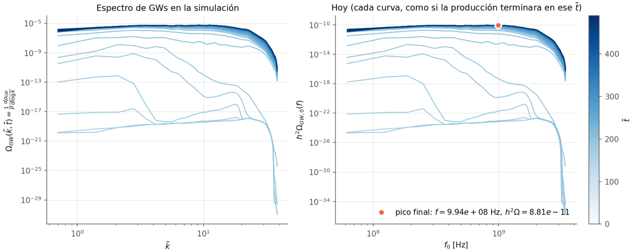
Figura 4: Monomial de control ( \phi^4 ), N = 64 . Espectro de GWs en la red (izquierda) y llevado a hoy (derecha), a cada tiempo de salida (claro = temprano).
