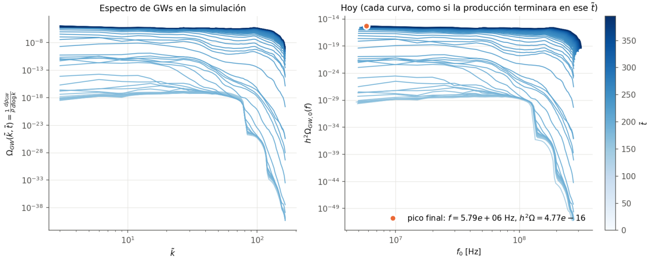
Figura 6: Monomial cuadrático de control ( m^2\phi^2/2 ), N = 64 . Espectro de GWs en la red (izquierda) y llevado a hoy con T_{RH} = 10^{10} GeV y w = 0 hasta el reheating (derecha), a cada tiempo de salida (claro = temprano).
