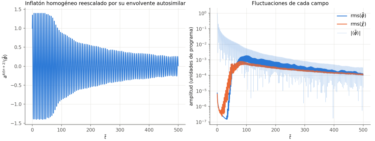
Figura 3: Monomial de control ( \phi^4 ), N = 64 . Izquierda: \langle\tilde{\phi}\rangle multiplicado por a^{6/(n+2)} = a , que sería una oscilación de amplitud constante sin resonancia. Derecha: rms de cada campo y |\langle\tilde{\phi}\rangle| .
