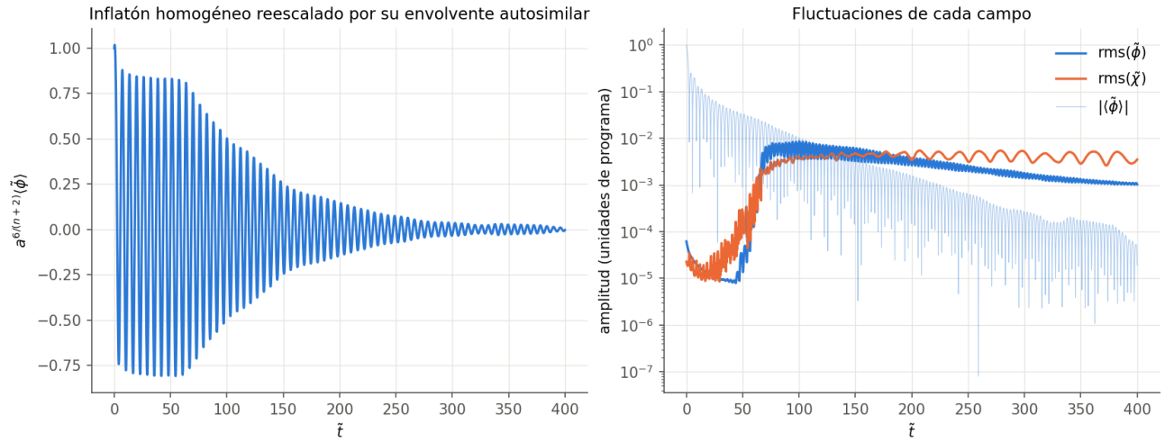
Figura 7: E-model cuadrático (Starobinsky), \alpha_K = 1 , N = 64 . Izquierda: \langle \tilde{\phi} \rangle multiplicado por a^{6/(n+2)} = a^{3/2} , que sin resonancia oscilaría con amplitud constante. Derecha: rms de cada campo y |\langle \tilde{\phi} \rangle| .
