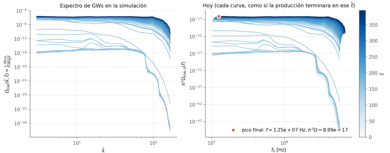
Figura 8: E-model cuadrático (Starobinsky), \alpha_K = 1 , N = 64 . Espectro de GWs en la red (izquierda) y llevado a hoy con T_{RH} = 10^{10} GeV y w = 0 hasta el reheating (derecha), a cada tiempo de salida (claro = temprano).
