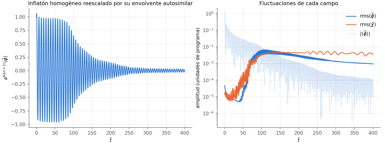
Figura 9: E-model cuadrático, \alpha_K = 5 , N = 64 . Izquierda: \langle \tilde{\phi} \rangle multiplicado por a^{6/(n+2)} = a^{3/2} , que sin resonancia oscilaría con amplitud constante. Derecha: rms de cada campo y |\langle \tilde{\phi} \rangle| .
