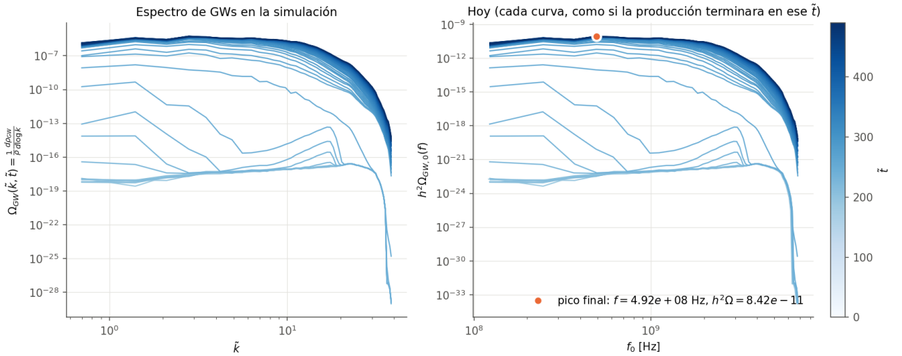
Figura 6: E-model, \alpha_K = 5 , N = 64 . Espectro de GWs en la red (izquierda) y llevado a hoy (derecha), a cada tiempo de salida (claro = temprano).
