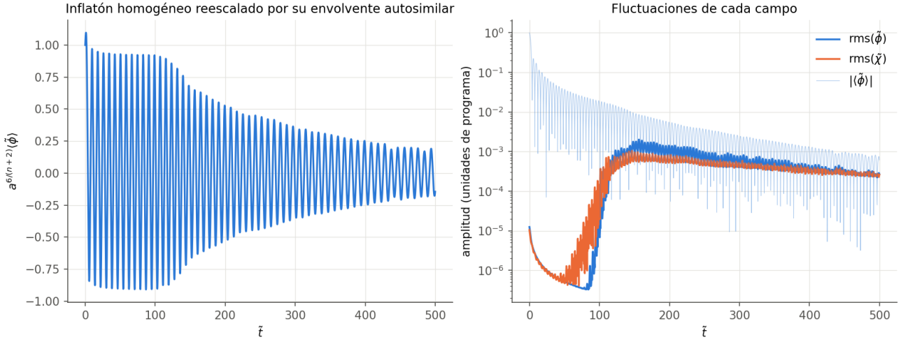
Figura 5: E-model, \alpha_K = 5 , N = 64 . Izquierda: \langle \tilde{\phi} \rangle multiplicado por a^{6/(n+2)} = a , que sería una oscilación de amplitud constante sin resonancia. Derecha: rms de cada campo y |\langle \tilde{\phi} \rangle| .
