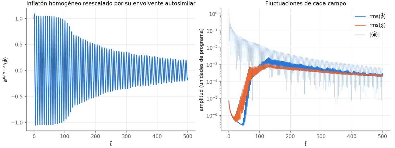
Figura 3: T-model, \alpha_K = 1 , N = 64 . Izquierda: \langle\tilde{\phi}\rangle multiplicado por a^{6/(n+2)} = a , que sería una oscilación de amplitud constante sin resonancia. Derecha: rms de cada campo y |\langle\tilde{\phi}\rangle| .
