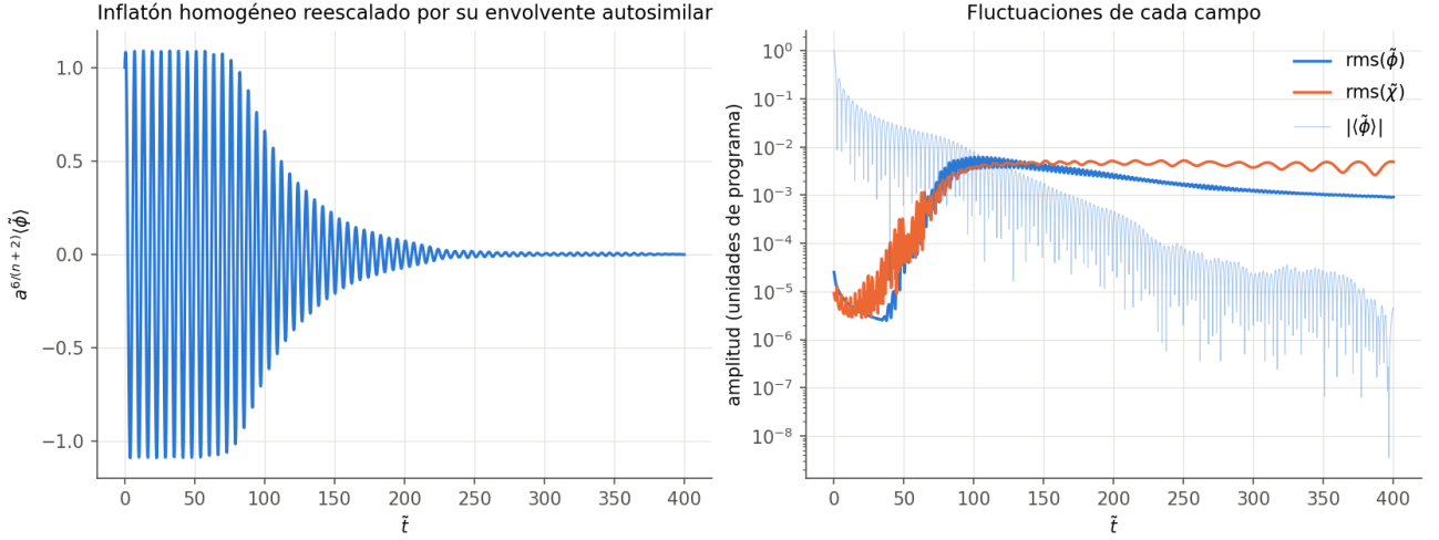
Figura 5: T-model cuadrático, \alpha_K = 1 , N = 64 . Izquierda: \langle \tilde{\phi} \rangle multiplicado por a^{6/(n+2)} = a^{3/2} , que sin resonancia oscilaría con amplitud constante. Derecha: rms de cada campo y |\langle \tilde{\phi} \rangle| .
