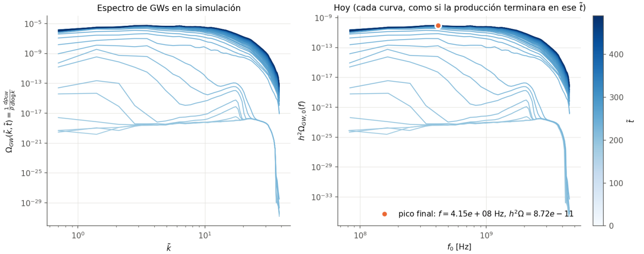
Figura 4: T-model, \alpha_K = 1 , N = 64 . Espectro de GWs en la red (izquierda) y llevado a hoy (derecha), a cada tiempo de salida (claro = temprano).
