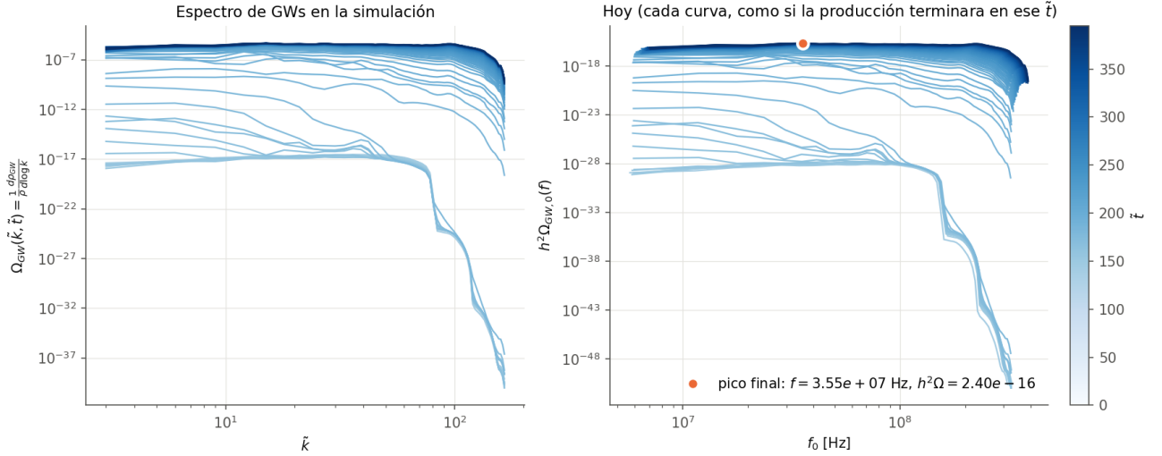
Figura 6: T-model cuadrático, \alpha_K = 1 , N = 64 . Espectro de GWs en la red (izquierda) y llevado a hoy con T_{RH} = 10^{10} GeV y w = 0 hasta el reheating (derecha), a cada tiempo de salida (claro = temprano).
