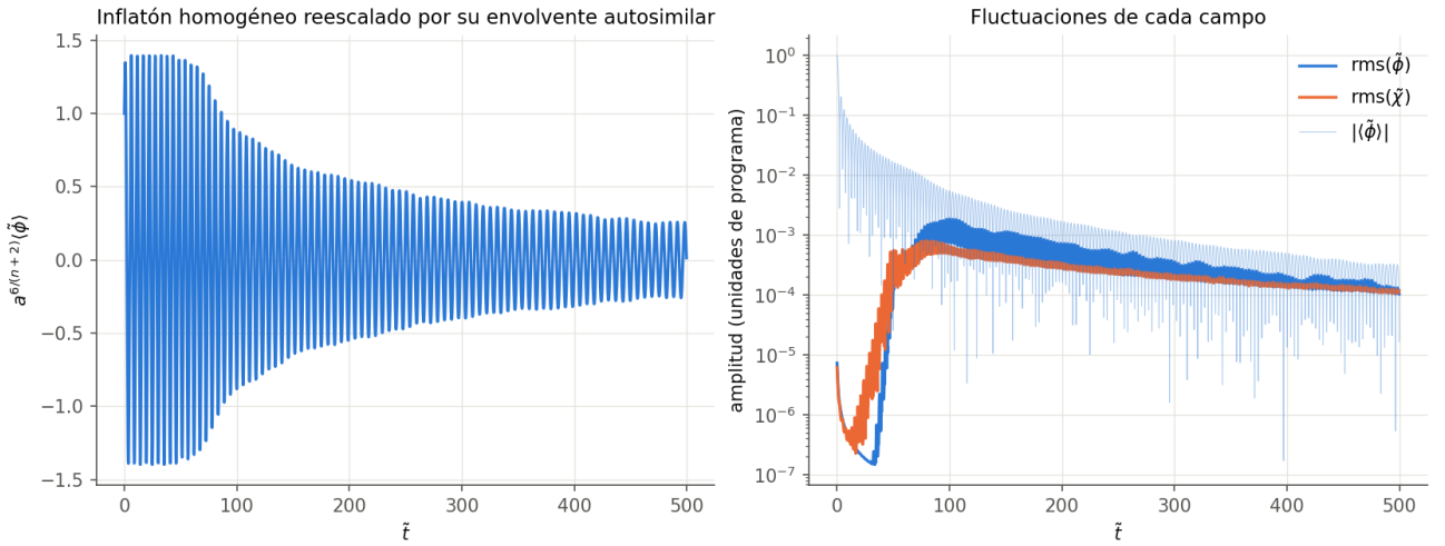
Figura 5: Monomial de control ( \phi^4 ), N = 64 . Izquierda: \langle \tilde{\phi} \rangle multiplicado por a^{6/(n+2)} = a , que sería una oscilación de amplitud constante sin resonancia. Derecha: rms de cada campo y |\langle \tilde{\phi} \rangle| .
