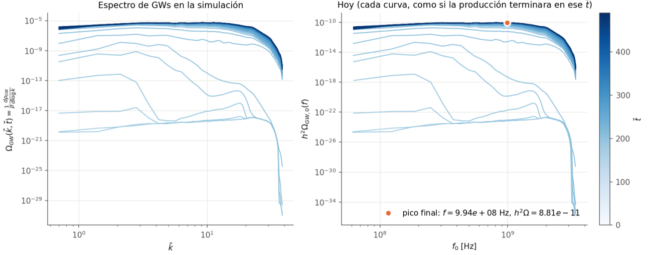
Figura 6: Monomial de control ( \phi^4 ), N = 64 . Espectro de GWs en la red (izquierda) y llevado a hoy (derecha), a cada tiempo de salida (claro = temprano).
