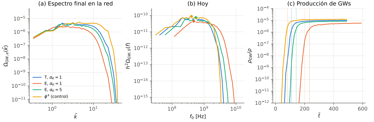
Figura 2: Los cuatro casos cuárticos con N = 128 , \tilde{k}_{\text{IR}} = 0,35 y la misma semilla. Paneles como en la Fig. 1.
