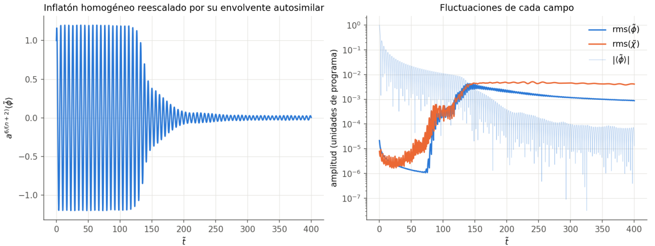
Figura 7: Monomial cuadrático de control ( m^2 \phi^2/2 ), N = 64 . Izquierda: \langle \tilde{\phi} \rangle multiplicado por a^{6/(n+2)} = a^{3/2} , que sin resonancia oscilaría con amplitud constante. Derecha: rms de cada campo y |\langle \tilde{\phi} \rangle| .
