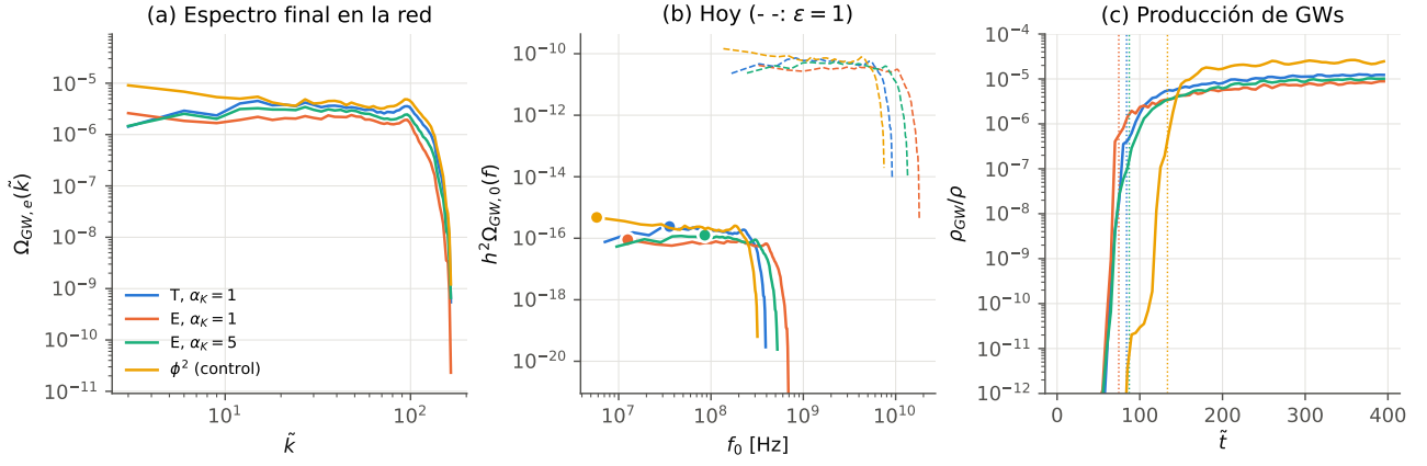
Figura 3: Los cuatro casos cuadráticos con N = 64 y la misma semilla. (a) Espectro de GWs al final de la simulación. (b) Llevado a hoy con T_{RH} = 10^{10} GeV y w = 0 hasta el reheating (línea llena; el punto marca el máximo), y con \epsilon = 1 , radiación desde el final de la simulación (línea cortada). (c) Fracción de la energía en GWs; la línea punteada marca cuándo \text{rms}(\tilde{\chi}) llega a la mitad de su máximo.
