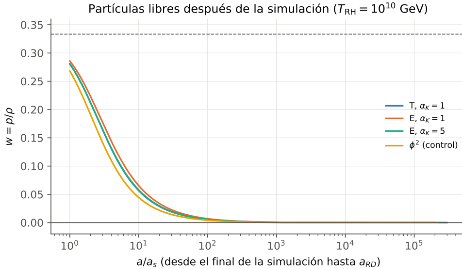
Figura 4: w(a) entre el final de la simulación ( a_s ) y el reheating ( T_{\text{RH}} = 10^{10} GeV, a_{\text{RD}} \simeq 2\text{--}3 \times 10^5 a_s ), en el modelo de partículas libres con masas de campo medio. La línea de trazos es w = 1/3 .
