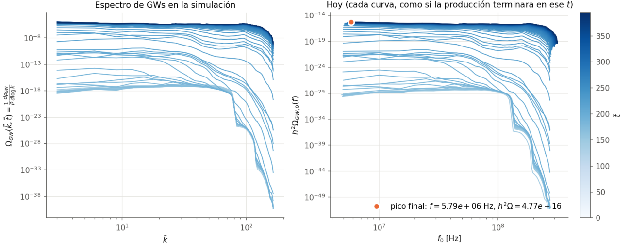
Figura 6: Monomial cuadrático de control ( m^2\phi^2/2 ), N = 64 . Espectro de GWs en la red (izquierda) y llevado a hoy con T_{\text{RH}} = 10^{10} GeV y w = 0 hasta el reheating (derecha), a cada tiempo de salida (claro = temprano).
