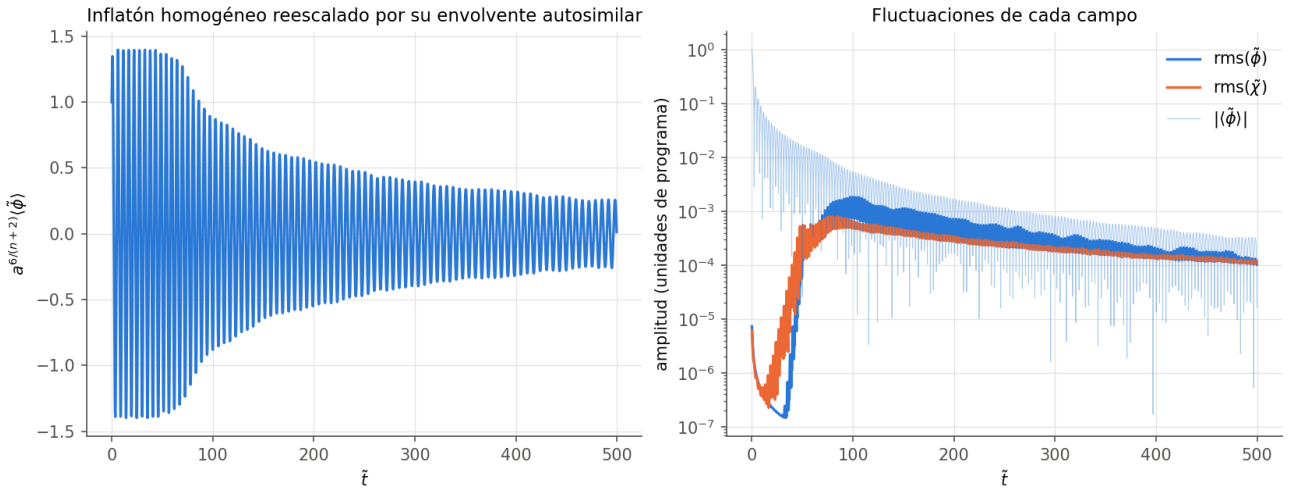
Figura 3: Monomial de control ( \phi^4 ), N = 64 . Izquierda: \langle\tilde{\phi}\rangle multiplicado por a^{6/(n+2)} = a , que sería una oscilación de amplitud constante sin resonancia. Derecha: rms de cada campo y |\langle\tilde{\phi}\rangle| .
