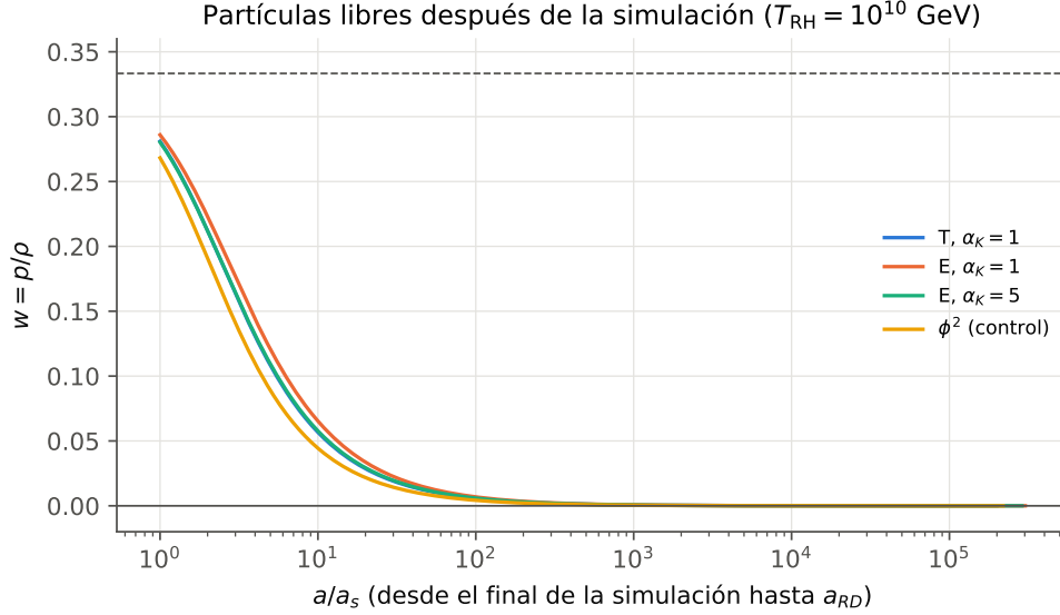
Figura 3: w(a) entre el final de la simulación ( a_s ) y el reheating ( T_{\text{RH}} = 10^{10} GeV, a_{\text{RD}} \simeq 2\text{--}3 \times 10^5 a_s ), en el modelo de partículas libres con masas de campo medio. La línea de trazos es w = 1/3 .
