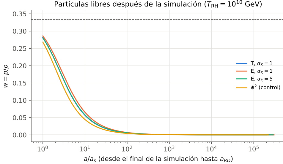
Figura 3: w(a) entre el final de la simulación ( a_s ) y el reheating ( T_{RH} = 10^{10} GeV, a_{RD} \simeq 2-3 \times 10^5 a_s ), en el modelo de partículas libres con masas de campo medio. La línea de trazos es w = 1/3 .
