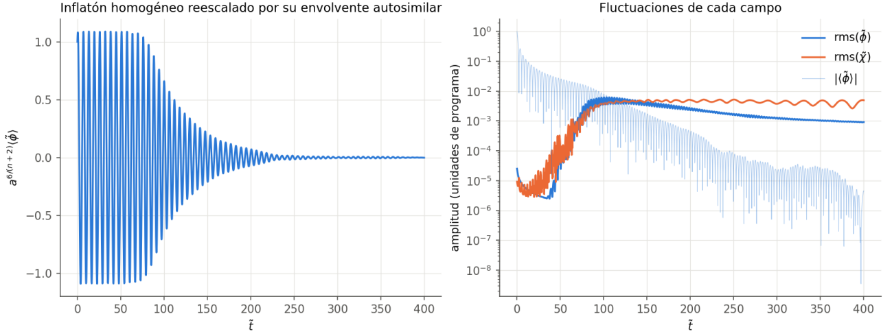
Figura 6: T-model cuadrático, \alpha_K = 1 , N = 64 . Izquierda: \langle \tilde{\phi} \rangle multiplicado por a^{6/(n+2)} = a^{3/2} , que sin resonancia oscilaría con amplitud constante. Derecha: rms de cada campo y |\langle \tilde{\phi} \rangle| .
