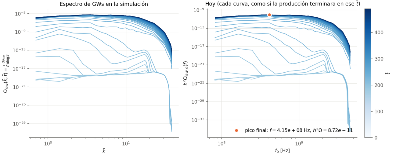
Figura 5: T-model, \alpha_K = 1 , N = 64 . Espectro de GWs en la red (izquierda) y llevado a hoy (derecha), a cada tiempo de salida (claro = temprano).
