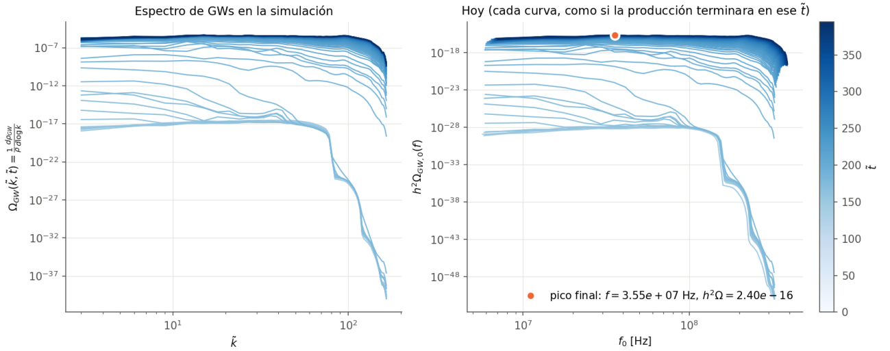
Figura 7: T-model cuadrático, \alpha_K = 1 , N = 64 . Espectro de GWs en la red (izquierda) y llevado a hoy con T_{RH} = 10^{10} GeV y w = 0 hasta el reheating (derecha), a cada tiempo de salida (claro = temprano).
