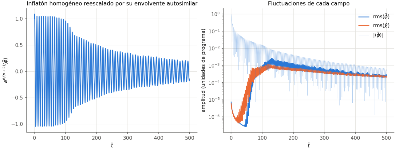
Figura 4: T-model, \alpha_K = 1 , N = 64 . Izquierda: \langle\tilde{\phi}\rangle multiplicado por a^{6/(n+2)} = a , que sería una oscilación de amplitud constante sin resonancia. Derecha: rms de cada campo y |\langle\tilde{\phi}\rangle| .
