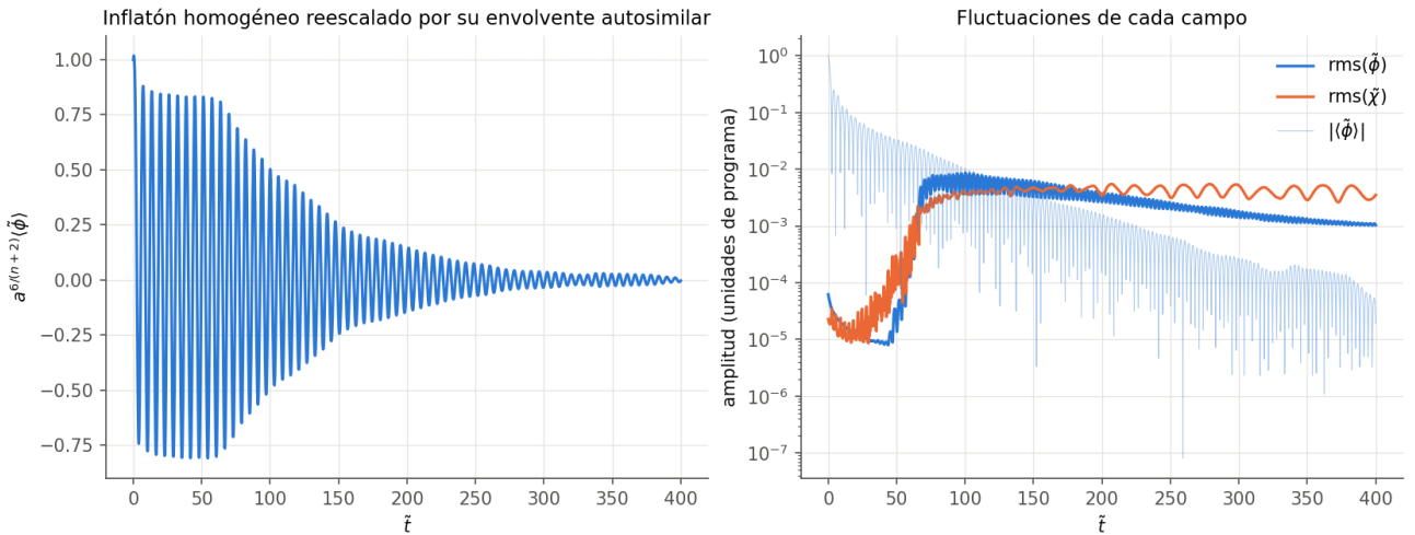
Figura 8: E-model cuadrático (Starobinsky), \alpha_K = 1 , N = 64 . Izquierda: \langle\tilde{\phi}\rangle multiplicado por a^{6/(n+2)} = a^{3/2} , que sin resonancia oscilaría con amplitud constante. Derecha: rms de cada campo y |\langle\tilde{\phi}\rangle| .
