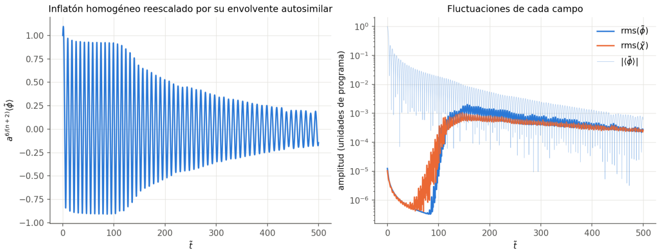
Figura 6: E-model, \alpha_K = 5 , N = 64 . Izquierda: \langle\tilde{\phi}\rangle multiplicado por a^{6/(n+2)} = a , que sería una oscilación de amplitud constante sin resonancia. Derecha: rms de cada campo y |\langle\tilde{\phi}\rangle| .
