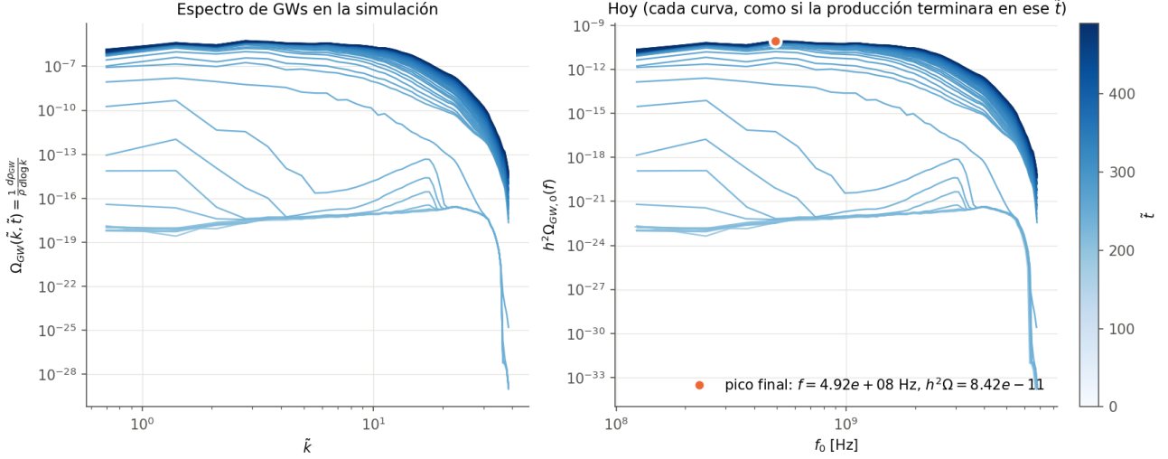
Figura 7: E-model, \alpha_K = 5 , N = 64 . Espectro de GWs en la red (izquierda) y llevado a hoy (derecha), a cada tiempo de salida (claro = temprano).
