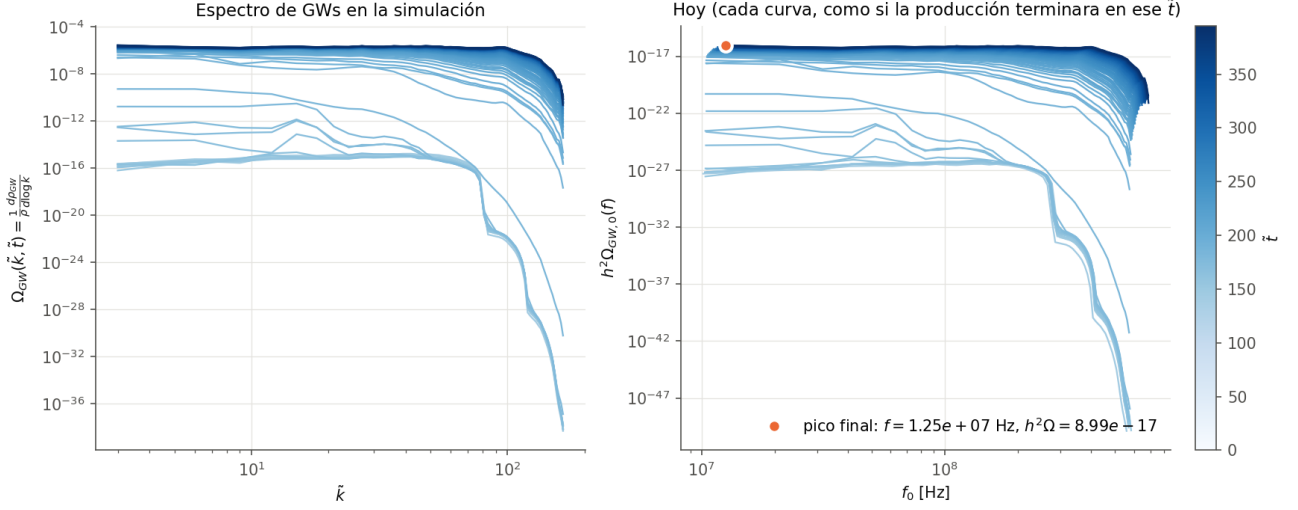
Figura 9: E-model cuadrático (Starobinsky), \alpha_K = 1 , N = 64 . Espectro de GWs en la red (izquierda) y llevado a hoy con T_{\text{RH}} = 10^{10} GeV y w = 0 hasta el reheating (derecha), a cada tiempo de salida (claro = temprano).
