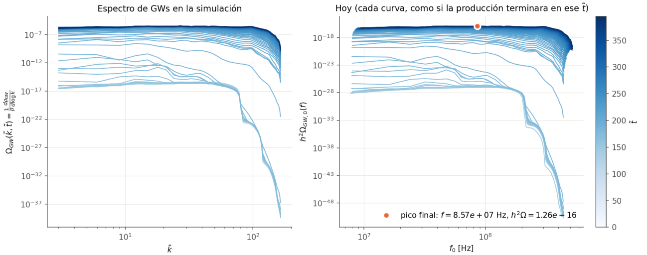
Figura 11: E-model cuadrático, \alpha_K = 5 , N = 64 . Espectro de GWs en la red (izquierda) y llevado a hoy con T_{\text{RH}} = 10^{10} GeV y w = 0 hasta el reheating (derecha), a cada tiempo de salida (claro = temprano).
