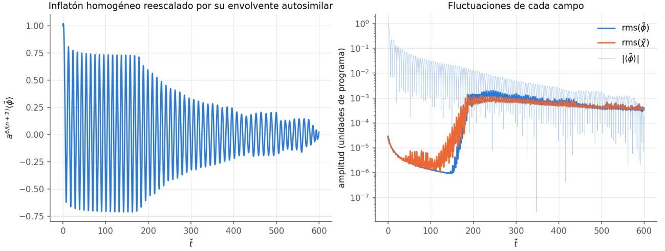
Figura 4: E-model, \alpha_K = 1 , N = 64 . Izquierda: \langle\tilde{\phi}\rangle multiplicado por a^{6/(n+2)} = a , que sería una oscilación de amplitud constante sin resonancia. Derecha: rms de cada campo y |\langle\tilde{\phi}\rangle| .
