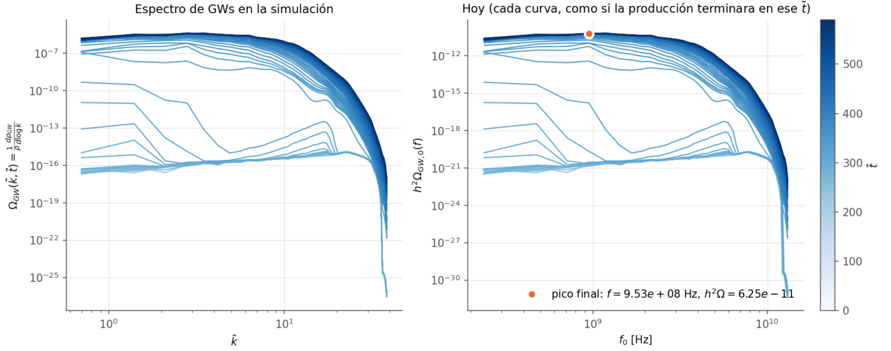
Figura 5: E-model, \alpha_K = 1 , N = 64 . Espectro de GWs en la red (izquierda) y llevado a hoy (derecha), a cada tiempo de salida (claro = temprano). La corrida llega a \tilde{t} = 600 .
