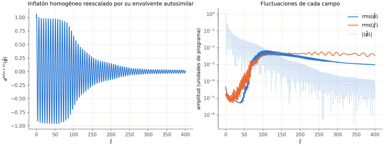
Figura 10: E-model cuadrático, \alpha_K = 5 , N = 64 . Izquierda: \langle \tilde{\phi} \rangle multiplicado por a^{6/(n+2)} = a^{3/2} , que sin resonancia oscilaría con amplitud constante. Derecha: rms de cada campo y |\langle \tilde{\phi} \rangle| .
