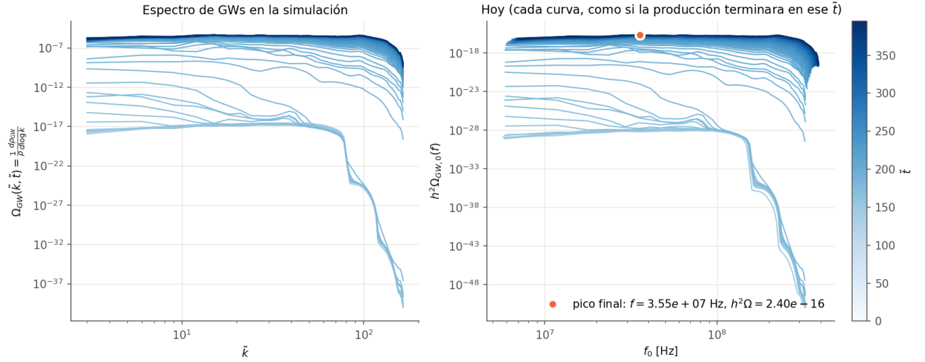
Figura 8: T-model cuadrático, \alpha_K = 1 , N = 64 . Espectro de GWs en la red (izquierda) y llevado a hoy con T_{\text{RH}} = 10^{10} GeV y w = 0 hasta el reheating (derecha), a cada tiempo de salida (claro = temprano).
