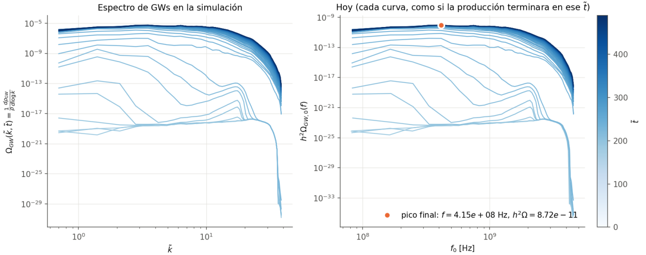
Figura 6: T-model, \alpha_K = 1 , N = 64 . Espectro de GWs en la red (izquierda) y llevado a hoy (derecha), a cada tiempo de salida (claro = temprano).
