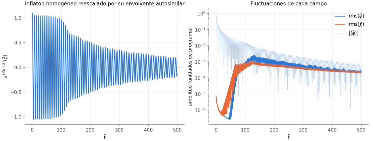
Figura 5: T-model, \alpha_K = 1 , N = 64 . Izquierda: \langle \tilde{\phi} \rangle multiplicado por a^{6/(n+2)} = a , que sería una oscilación de amplitud constante sin resonancia. Derecha: rms de cada campo y |\langle \tilde{\phi} \rangle| .
