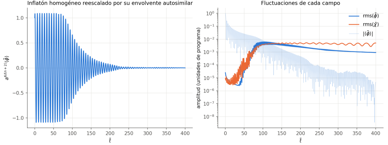
Figura 7: T-model cuadrático, \alpha_K = 1 , N = 64 . Izquierda: \langle\tilde{\phi}\rangle multiplicado por a^{6/(n+2)} = a^{3/2} , que sin resonancia oscilaría con amplitud constante. Derecha: rms de cada campo y |\langle\tilde{\phi}\rangle| .
