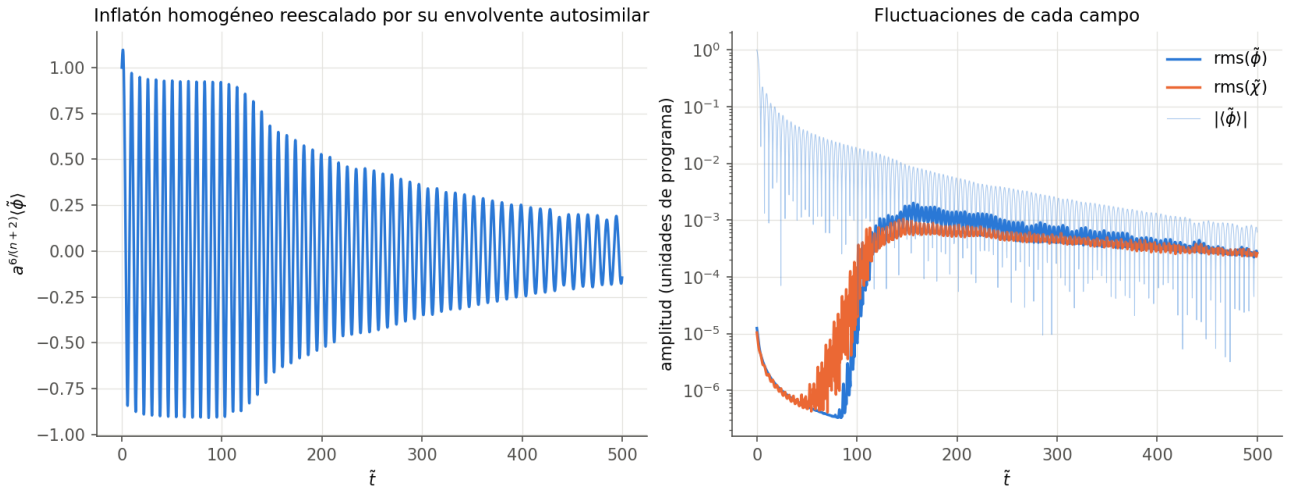
Figura 4: E-model, \alpha_K = 5 , N = 64 . Izquierda: \langle \tilde{\phi} \rangle multiplicado por a^{6/(n+2)} = a , que sería una oscilación de amplitud constante sin resonancia. Derecha: rms de cada campo y |\langle \tilde{\phi} \rangle| .
