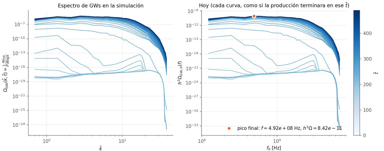
Figura 5: E-model, \alpha_K = 5 , N = 64 . Espectro de GWs en la red (izquierda) y llevado a hoy (derecha), a cada tiempo de salida (claro = temprano).
