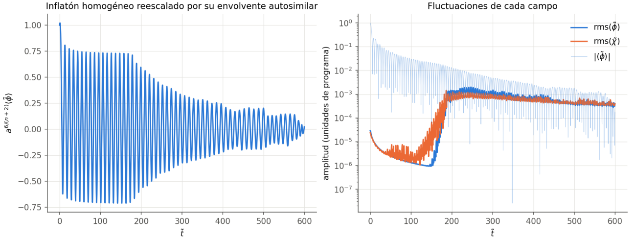
Figura 2: E-model, \alpha_K = 1 , N = 64 . Izquierda: \langle \tilde{\phi} \rangle multiplicado por a^{6/(n+2)} = a , que sería una oscilación de amplitud constante sin resonancia. Derecha: rms de cada campo y |\langle \tilde{\phi} \rangle| .
