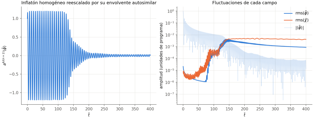
Figura 6: Monomial cuadrático de control ( m^2\phi^2/2 ), N = 64 . Izquierda: \langle\tilde{\phi}\rangle multiplicado por a^{6/(n+2)} = a^{3/2} , que sin resonancia oscilaría con amplitud constante. Derecha: rms de cada campo y |\langle\tilde{\phi}\rangle| .
