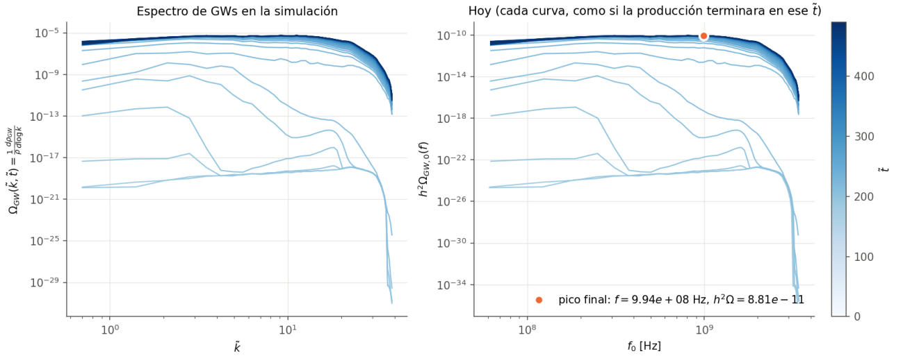
Figura 5: Monomial de control ( \phi^4 ), N = 64 . Espectro de GWs en la red (izquierda) y llevado a hoy (derecha), a cada tiempo de salida (claro = temprano).
