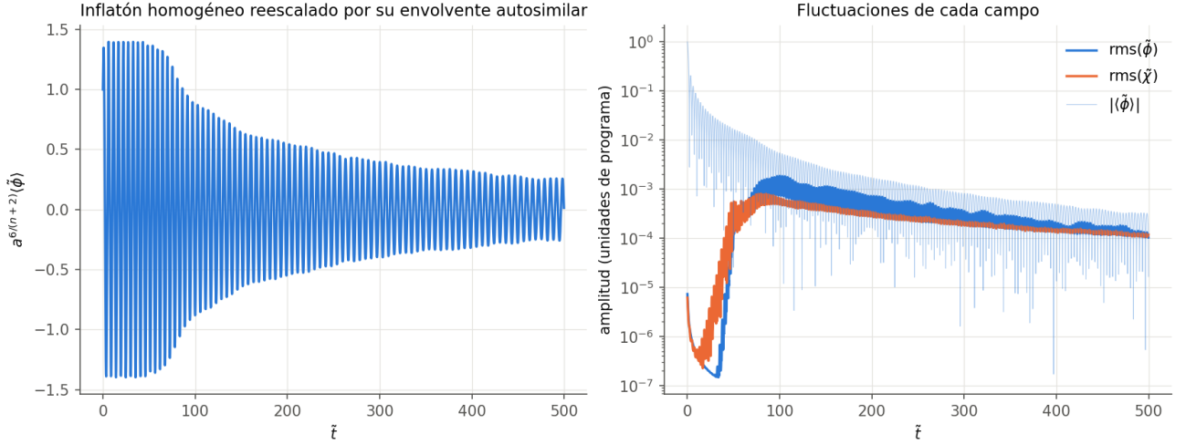
Figura 4: Monomial de control ( \phi^4 ), N = 64 . Izquierda: \langle\tilde{\phi}\rangle multiplicado por a^{6/(n+2)} = a , que sería una oscilación de amplitud constante sin resonancia. Derecha: rms de cada campo y |\langle\tilde{\phi}\rangle| .
