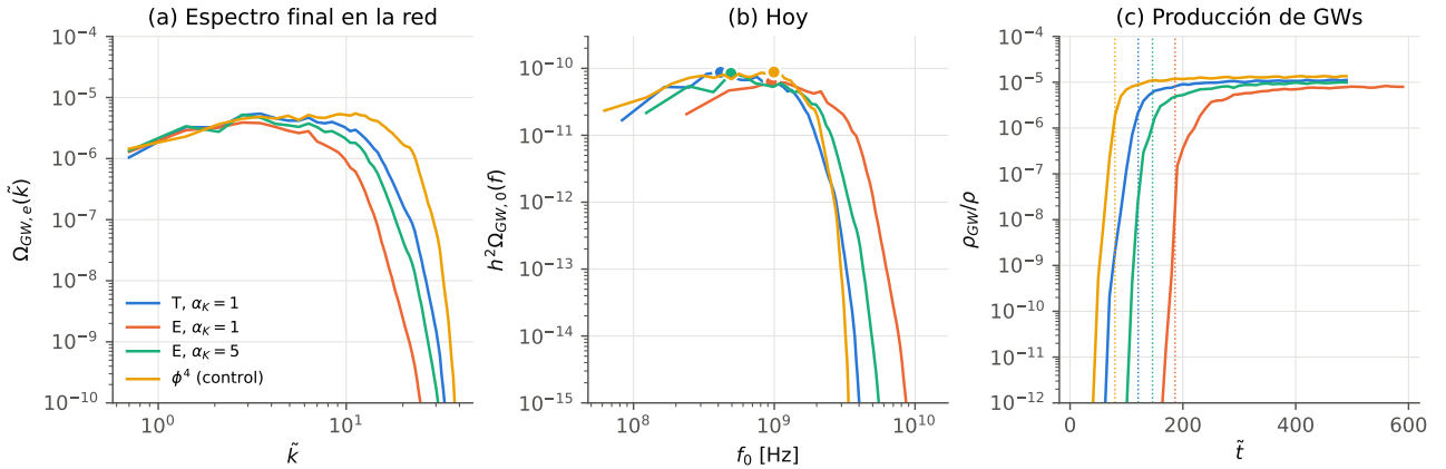
Figura 1: Los cuatro casos cuárticos con N = 64 . (a) Espectro de GWs al final de la simulación, en unidades de programa. (b) El mismo espectro llevado a hoy (Sec. 3.4); el punto marca el máximo. (c) Fracción de la energía en GWs; la línea punteada marca el máximo de \text{rms}(\tilde{\chi}) , es decir, cuándo la resonancia satura.
