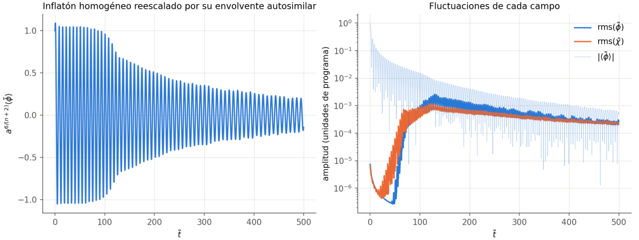
Figura 3: T-model, \alpha_K = 1 , N = 64 . Izquierda: \langle \tilde{\phi} \rangle multiplicado por a^{6/(n+2)} = a , que sería una oscilación de amplitud constante sin resonancia. Derecha: rms de cada campo y |\langle \tilde{\phi} \rangle| .
