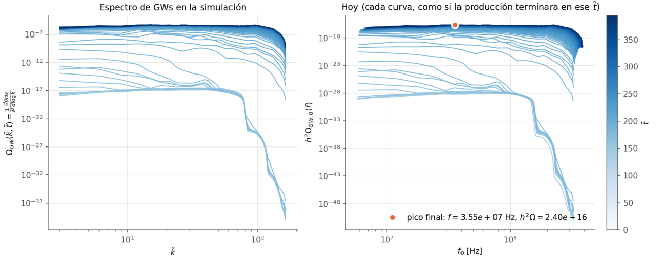
Figura 6: T-model cuadrático, \alpha_K = 1 , N = 64 . Espectro de GWs en la red (izquierda) y llevado a hoy con T_{\text{RH}} = 10^{10} GeV y w = 0 hasta el reheating (derecha), a cada tiempo de salida (claro = temprano).
