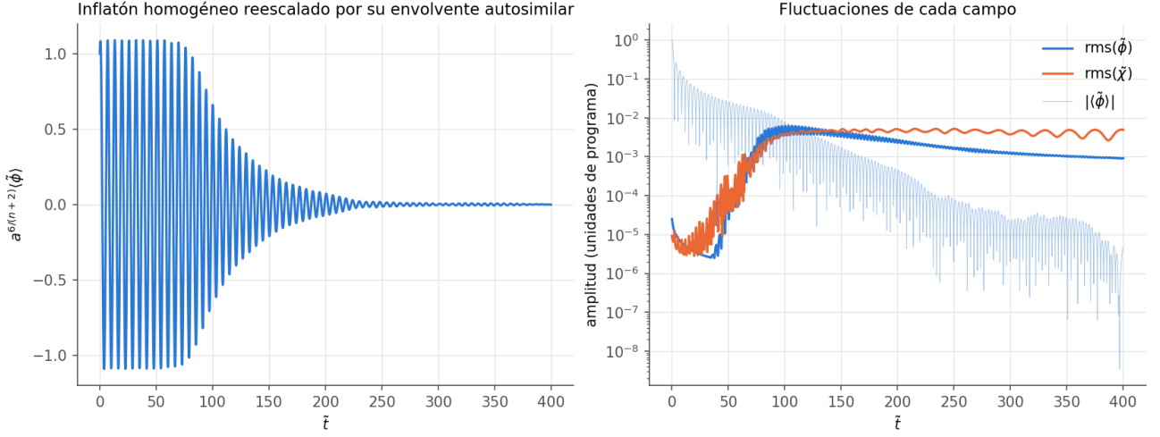
Figura 5: T-model cuadrático, \alpha_K = 1 , N = 64 . Izquierda: \langle\tilde{\phi}\rangle multiplicado por a^{6/(n+2)} = a^{3/2} , que sin resonancia oscilaría con amplitud constante. Derecha: rms de cada campo y |\langle\tilde{\phi}\rangle| .
