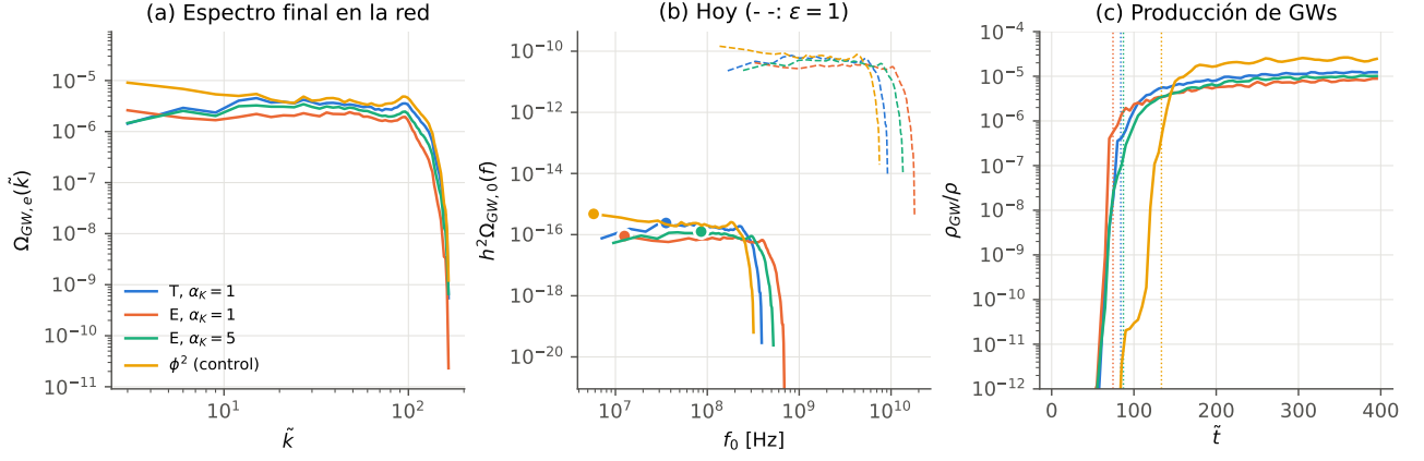
Figura 3: Los cuatro casos cuadráticos con N = 64 y la misma semilla. (a) Espectro de GWs al final de la simulación. (b) Llevado a hoy con T_{RH} = 10^{10} GeV y w = 0 hasta el reheating (línea llena; el punto marca el máximo), y con \epsilon = 1 , radiación desde el final de la simulación (línea cortada). (c) Fracción de la energía en GWs; la línea punteada marca cuándo \text{rms}(\tilde{\chi}) llega a la mitad de su máximo.
