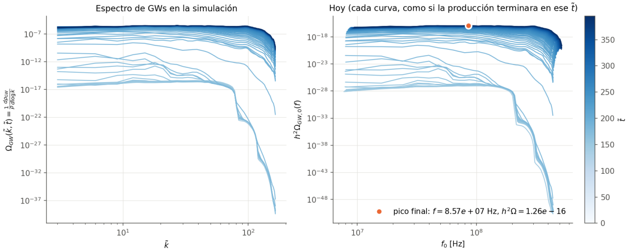
Figura 12: E-model cuadrático, \alpha_K = 5 , N = 64 . Espectro de GWs en la red (izquierda) y llevado a hoy con T_{RH} = 10^{10} GeV y w = 0 hasta el reheating (derecha), a cada tiempo de salida (claro = temprano).
