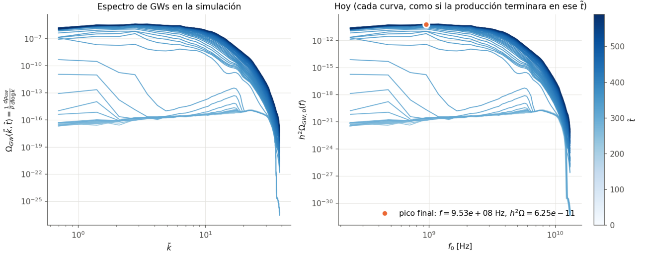
Figura 6: E-model, \alpha_K = 1 , N = 64 . Espectro de GWs en la red (izquierda) y llevado a hoy (derecha), a cada tiempo de salida (claro = temprano). La corrida llega a \tilde{t} = 600 .
