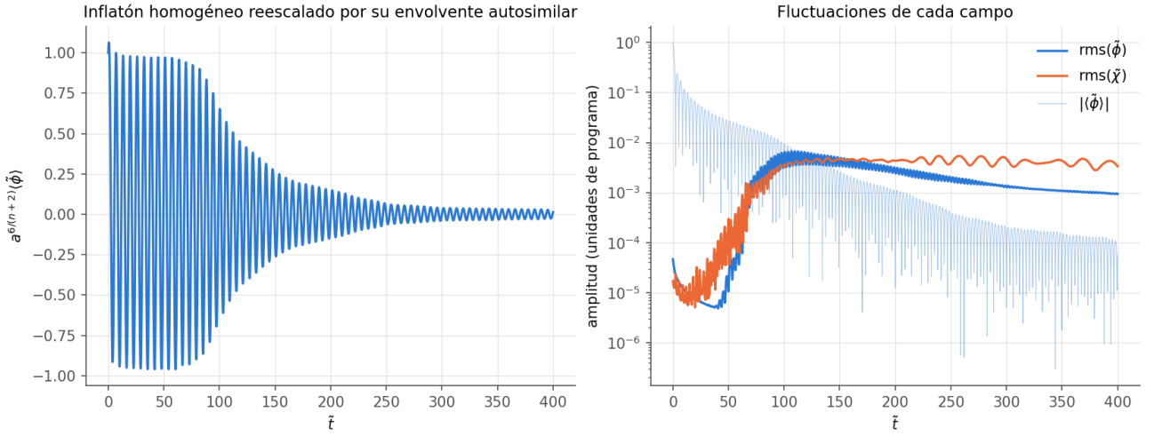
Figura 11: E-model cuadrático, \alpha_K = 5 , N = 64 . Izquierda: \langle \tilde{\phi} \rangle multiplicado por a^{6/(n+2)} = a^{3/2} , que sin resonancia oscilaría con amplitud constante. Derecha: rms de cada campo y |\langle \tilde{\phi} \rangle| .
