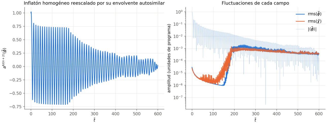
Figura 5: E-model, \alpha_K = 1 , N = 64 . Izquierda: \langle \tilde{\phi} \rangle multiplicado por a^{6/(n+2)} = a , que sería una oscilación de amplitud constante sin resonancia. Derecha: rms de cada campo y |\langle \tilde{\phi} \rangle| .
