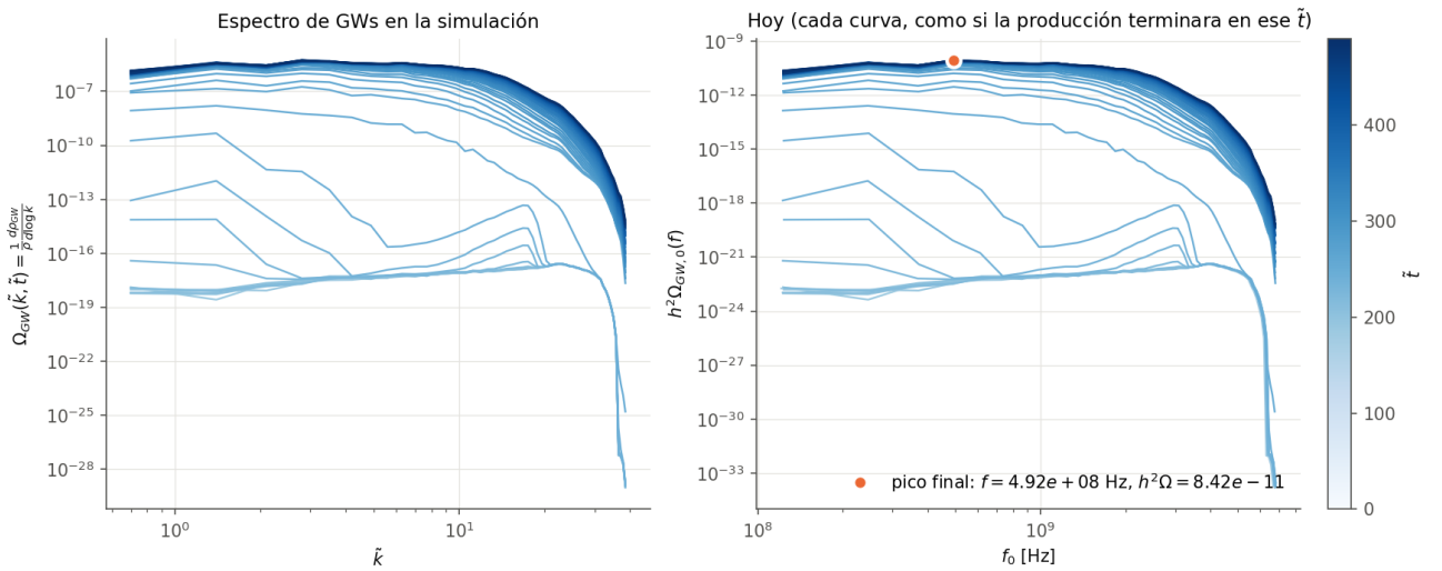
Figura 8: E-model, \alpha_K = 5 , N = 64 . Espectro de GWs en la red (izquierda) y llevado a hoy (derecha), a cada tiempo de salida (claro = temprano).
