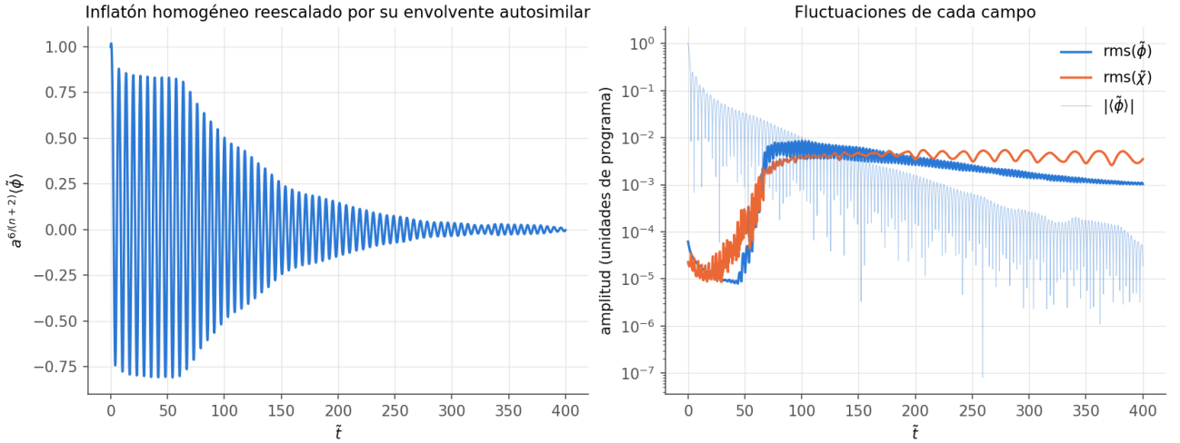
Figura 9: E-model cuadrático (Starobinsky), \alpha_K = 1 , N = 64 . Izquierda: \langle \tilde{\phi} \rangle multiplicado por a^{6/(n+2)} = a^{3/2} , que sin resonancia oscilaría con amplitud constante. Derecha: rms de cada campo y |\langle \tilde{\phi} \rangle| .
