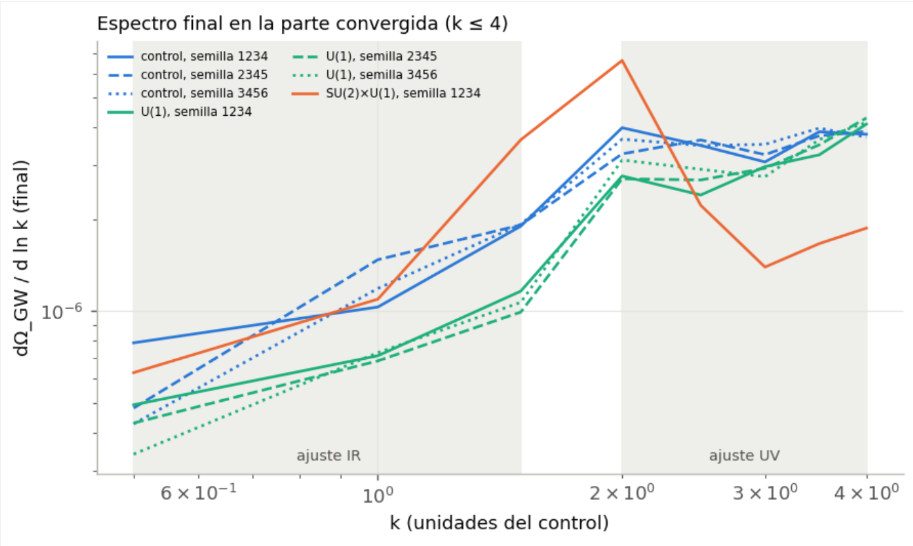
Espectro final en la parte confiable de las siete corridas (color: modelo; estilo de línea: semilla). Las franjas grises son las zonas de ajuste. Hecha con code/pendientes_espectro.py .
