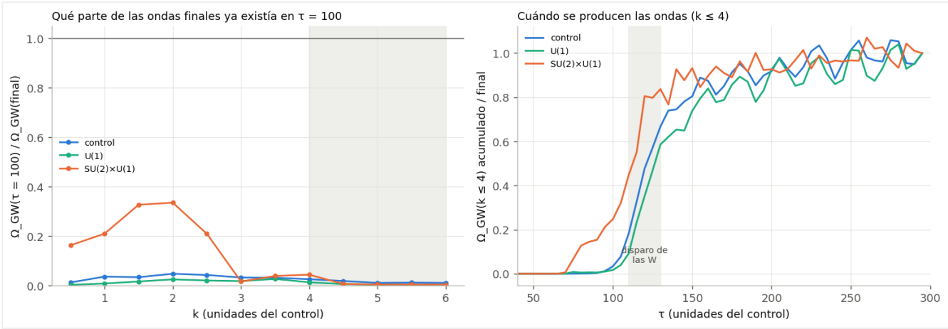
Izquierda: qué parte de las ondas finales ya existía en \tau = 100 , por k . Derecha: ondas acumuladas ( k \leq 4 ) contra el tiempo; la franja gris es el disparo de las W. Hecha con code/produccion_gws.py .
