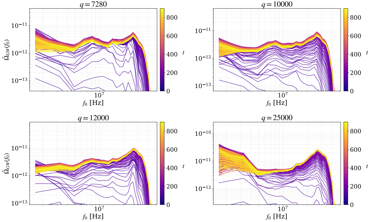
Figura 4.18: Espectro de ondas gravitacionales para el modelo m^2\phi^2 variando el parámetro de acoplamiento q . [Explicar mas]
