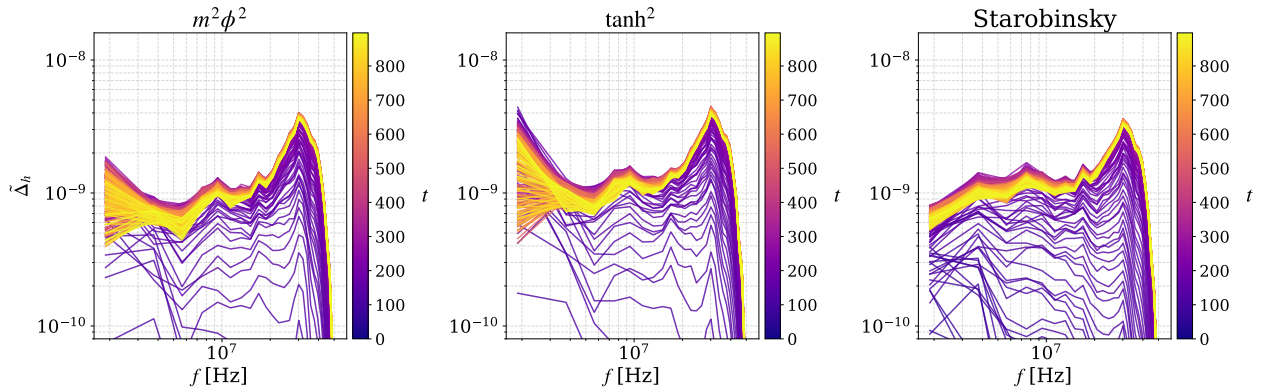
Figura 4.16: Espectro de potencias de las ondas gravitacionales proyectado a la actualidad para los modelos de tipo materia. Se aprecia una notable equivalencia morfológica y de amplitud entre los tres potenciales a escalas intermedias y ultravioletas. Las divergencias ruidosas en los modos infrarrojos constituyen artefactos numéricos de red originados por el volumen finito de la simulación. Los parámetros utilizados fueron m = 2,435 \times 10^{13} GeV, M = 2,435 \times 10^{19} GeV y \Lambda^4 = 1,7966 \times 10^{65} GeV 4 .
