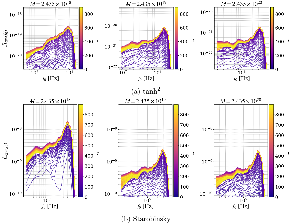
Figura 4.18: Espectro de ondas gravitacionales evaluado para distintos anchos de la meseta (parametrizados por M ) conservando la masa efectiva m constante de valor 1,46 \times 10^{13} GeV y el acoplamiento efectivo en q = 16000 . Mayores valores de M trasladan la potencia hacia modos ultravioletas y deprimen la señal estocástica total.
