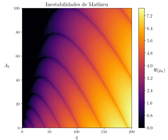
Figura 4: en esta imagen podemos ver cómo son las bandas para valores de q entre 0 y 200, y valores de A_k entre 0 y 100.
