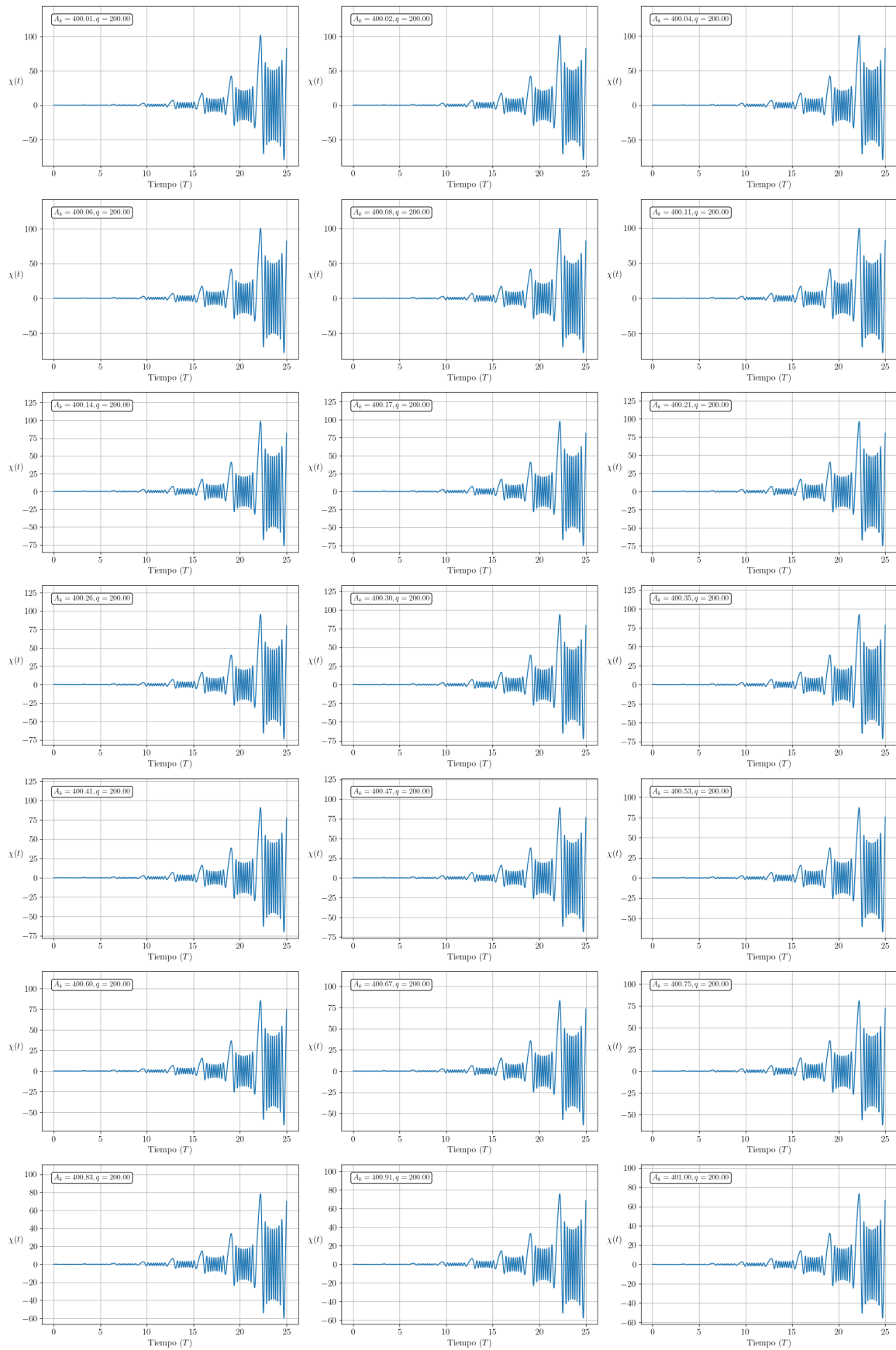
Figura 6: en esta imagen vemos cómo evolucionan las soluciones de la ecuación de Mathieu para distintos modos con q = 200 (broad resonance).
