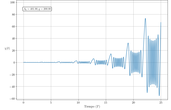
Figura 8: en esta imagen tenemos la evolución del modo con q = 200 y A_k = 401 lo que nos da una narrow resonance
