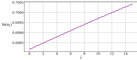
Figura 9: número de partículas para narrow resonance. Para esta figura tomamos q = 0,1 y A_k = 1,03 .
