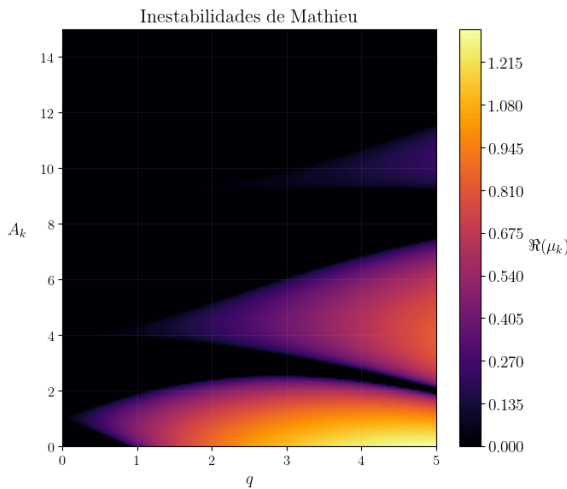
Figura 3: en esta imagen podemos ver cómo son las bandas para valores de q entre 0 y 5, y valores de A_k entre 0 y 15. Esta imagen es la misma que aparece en el texto de Mishra.
