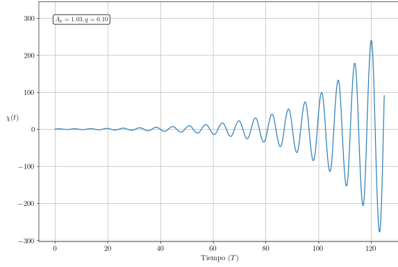
Figura 7: en esta imagen tenemos la evolución del modo con q = 0,1 y A_k = 1,03 lo que nos da una narrow resonance
