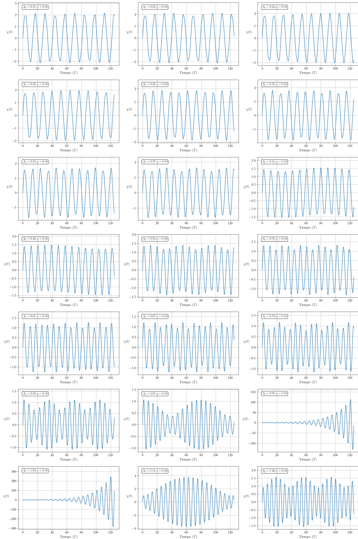
Figura 5: en esta imagen vemos cómo evolucionan las soluciones de la ecuación de Mathieu para distintos modos con q = 0,1 (narrow resonance).
