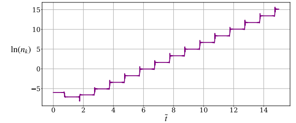
Figura 10: número de partículas para broad resonance. Para esta figura tomamos q = 200 y A_k = 401 .
