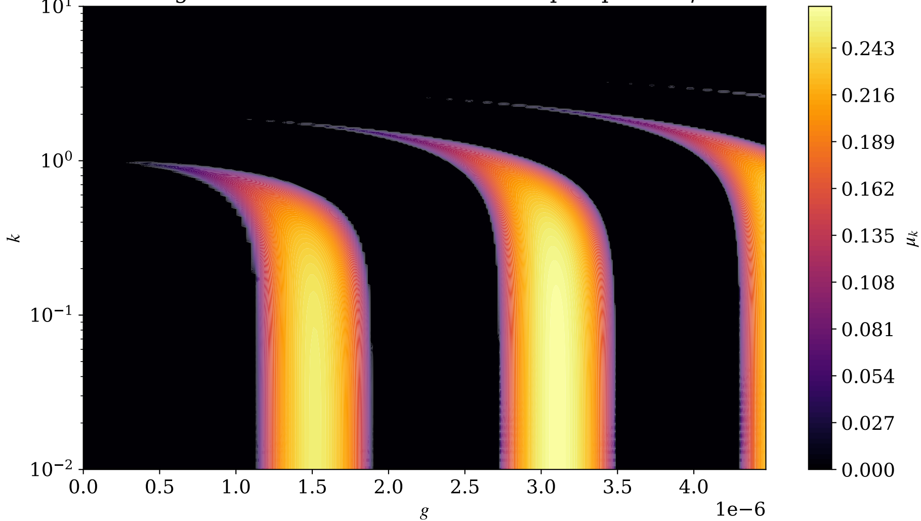
Diagrama de inestabilidades de Floquet para m^2\phi^2
