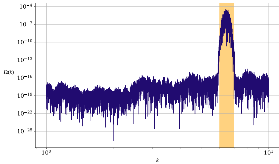
Figura 3.6: Espectro de potencia de las ondas gravitacionales calculado a partir de hacer un análisis lineal de la evolución de los campos. Se puede observar en la misma una zona sombreada de color naranja la cual representa la zona dónde el coeficiente de Floquet tiene parte real no nula y por tanto dónde se espera una amplificación como consecuencia de la resonancia paramétrica.
