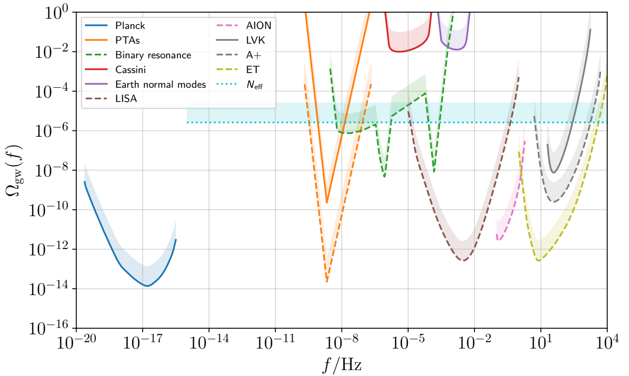
Figura 4.13: Sensibilidad de los detectores de ondas gravitacionales presentes y futuros junto con las cotas para la producción de éstas con los espectros observados con CosmoLattice superpuesto.
