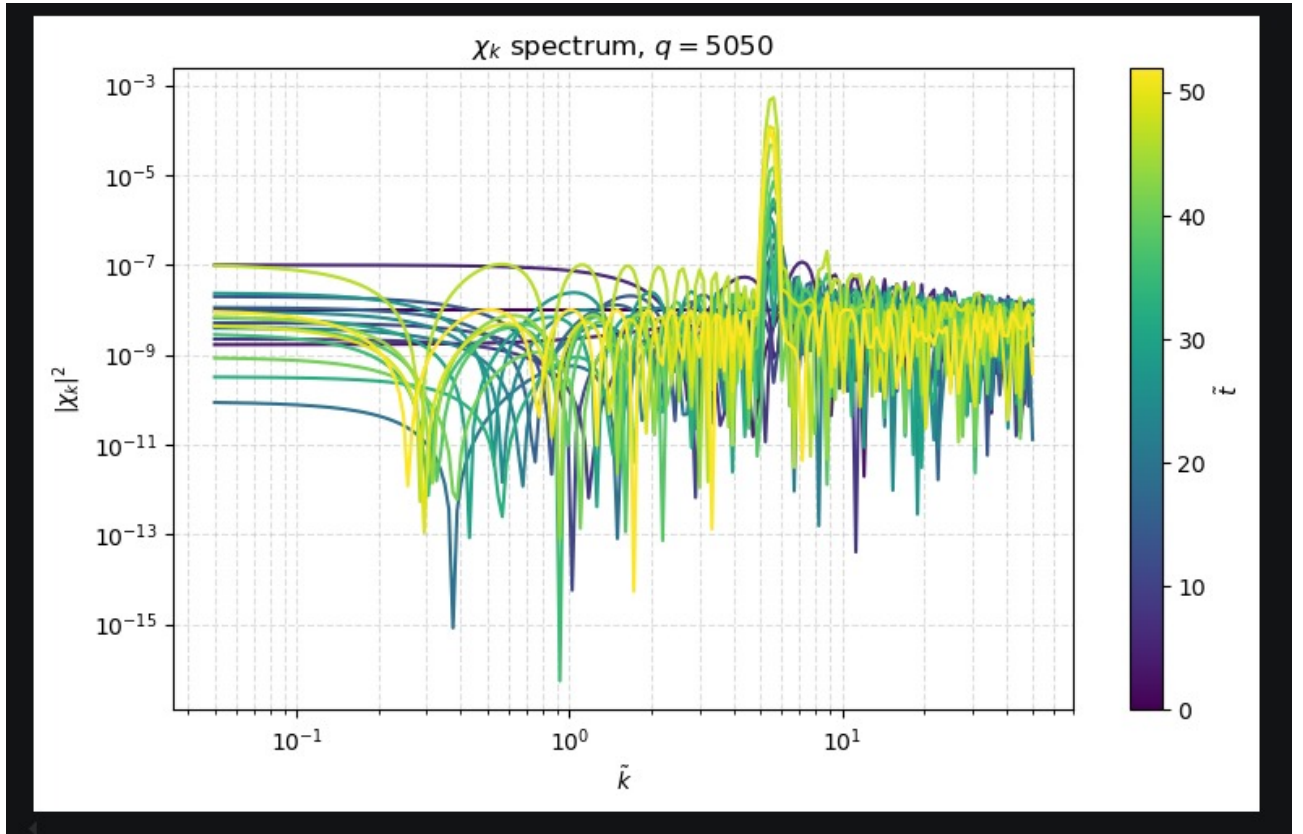
Figura 3.7: Evolución del espectro de potencias del campo hijo \mathcal{P}_\chi(k, \tau) . [AGREGAR DESCRIPCIÓN FÍSICA]
