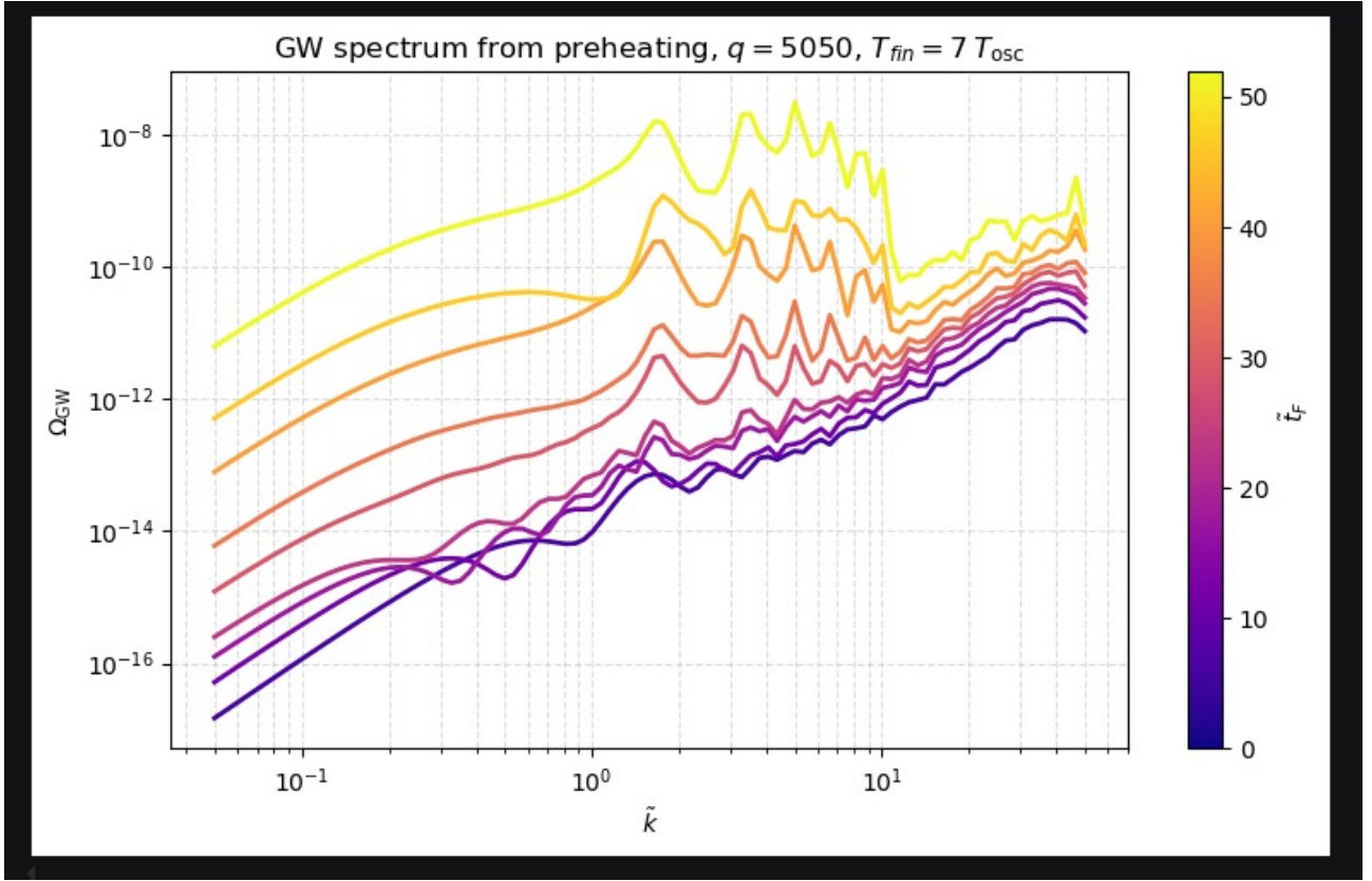
Figura 3.8: Evolución temporal del espectro de densidad de energía de las ondas gravitacionales \Omega_{GW} obtenida a partir del formalismo lineal. [AGREGAR DESCRIPCIÓN FÍSICA]
