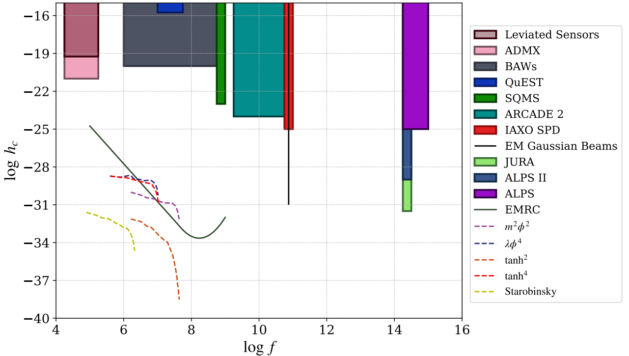
Figura 4.21: Deformación característica ( strain ) de las ondas gravitacionales generadas durante el reheating para los distintos modelos de inflatón estudiados. Las señales simuladas con \mathcal{CosmoLattice} se encuentran superpuestas a las curvas de sensibilidad de detectores estocásticos presentes y futuros (adaptado de [33]).
