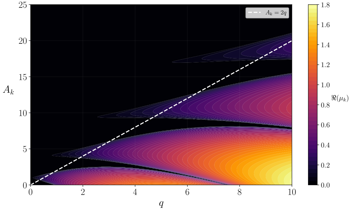
(a) m^2\phi^2
