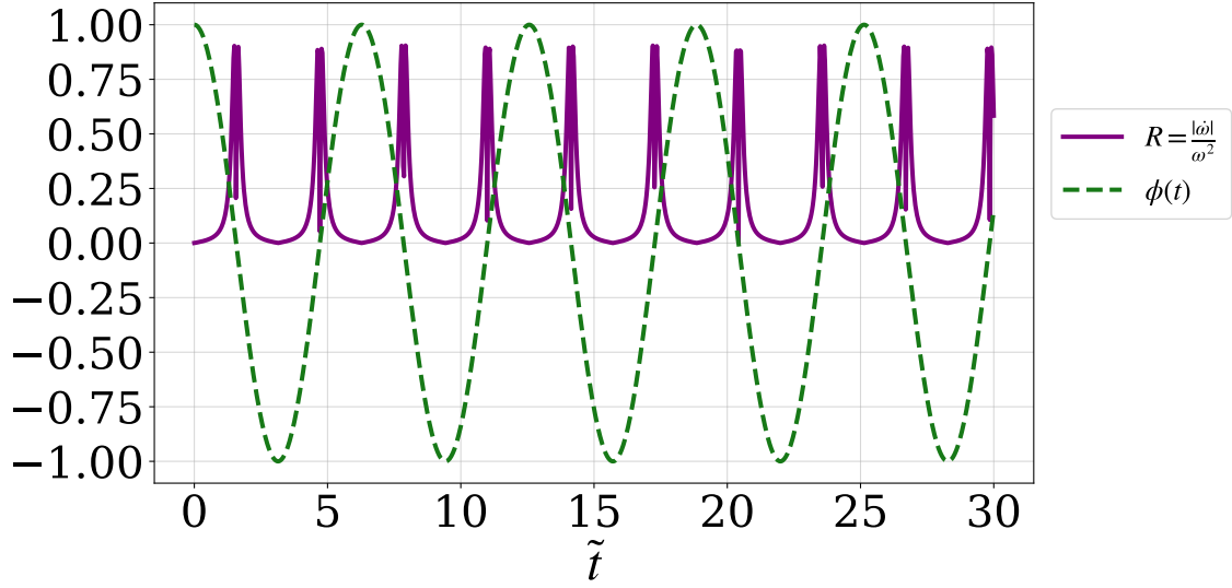
(a) m^2\phi^2
