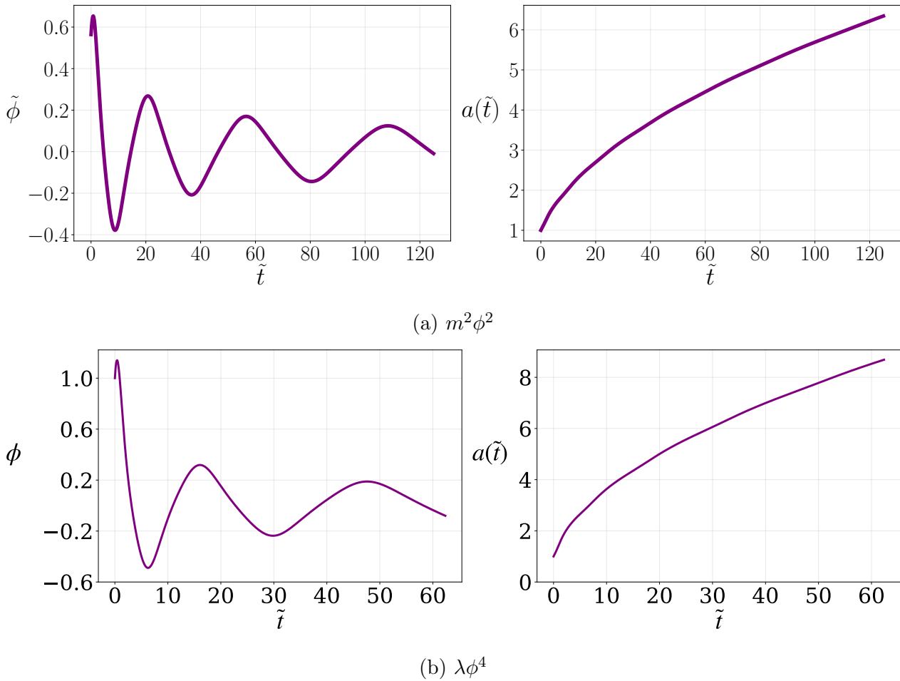
Figura 3.1: Evolución de la dinámica del background para cada modelo, donde se observa cómo el condensado del inflatón decae temporalmente mientras el factor de escala a(t) aumenta a un ritmo de (a) t^{2/3} y (b) t^{1/2} .
