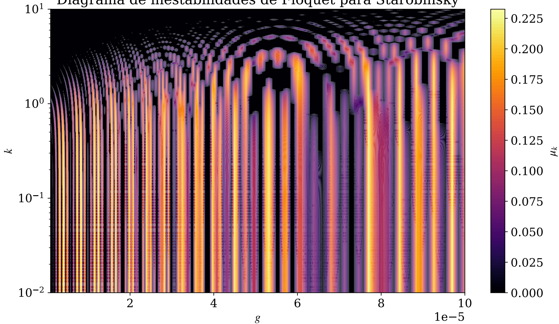
Diagrama de inestabilidades de Floquet para Starobinsky
