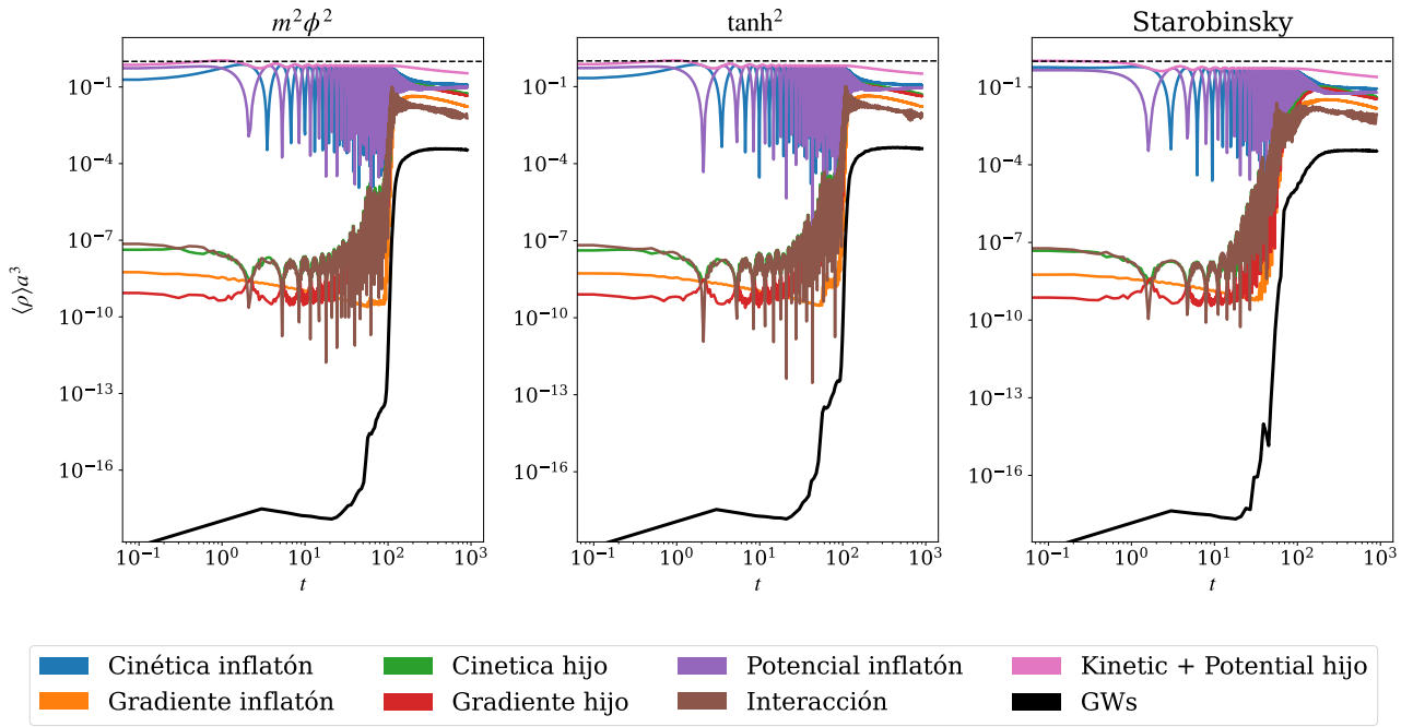
Figura 4.12: Evolución temporal de las densidades de energía para los campos de materia. Se comparan los modelos de tipo materia, evidenciando la sincronía entre el aumento de la energía de gradiente e interacción y el pico de producción de ondas gravitacionales.
