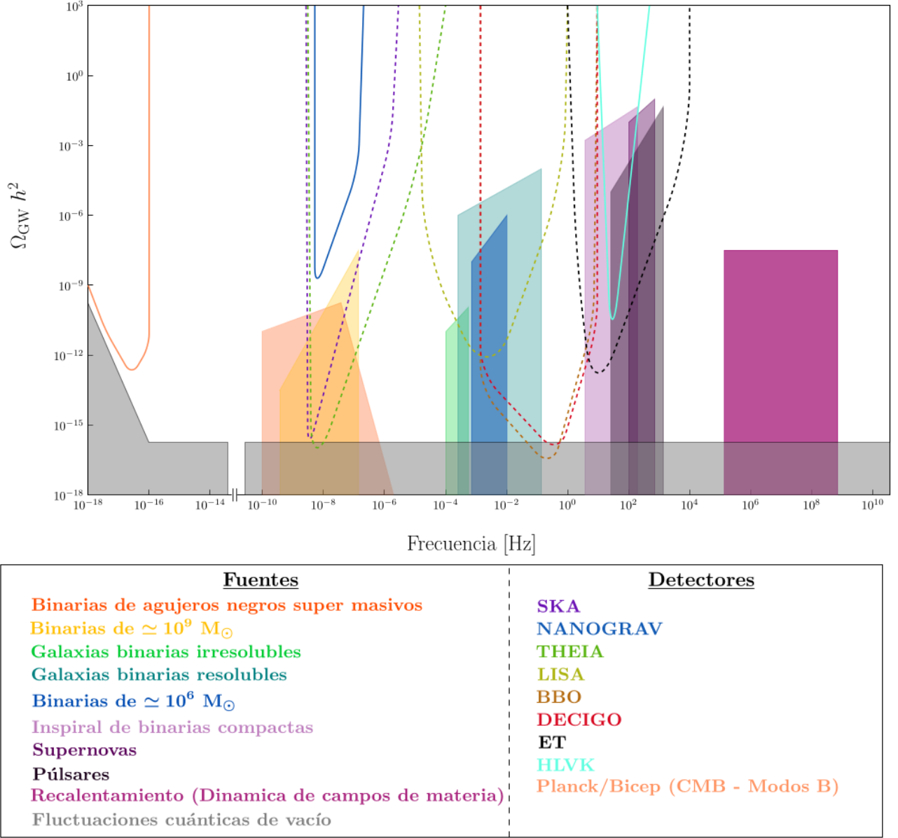
Figura 2.2: Bandas de frecuencias y densidad de energía de ondas gravitacionales esperado para diversos mecanismos astrofísicos y cosmológicos de producción de ondas gravitacionales. Además, se grafica en línea continua las curvas de sensibilidad para los detectores actualmente activos, mientras que en línea punteada las curvas de sensibilidad previstas para los detectores que al momento no se encuentran activos. Gráfico elaborado en base a [1, 12, 14, 36, 35].
