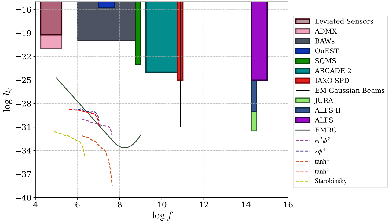
Figura 4.18: Deformación característica ( strain ) de las ondas gravitacionales generadas durante el preheating para los distintos modelos de inflatón estudiados. Las señales simuladas con CosmoLattice se encuentran superpuestas a las curvas de sensibilidad proyectadas para detectores estocásticos de ultra-alta frecuencia (adaptado de [43]).
