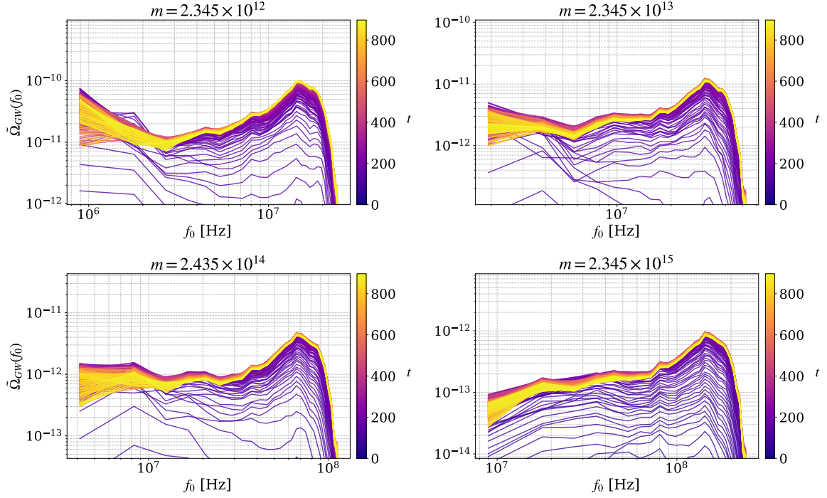
Figura 4.16: Espectro de potencias para el modelo m^2\phi^2 ante variaciones de la masa m . Masas más elevadas suprimen la amplitud espectral debido a una transferencia de energía acelerada que acorta la ventana de eficiencia resonante.
