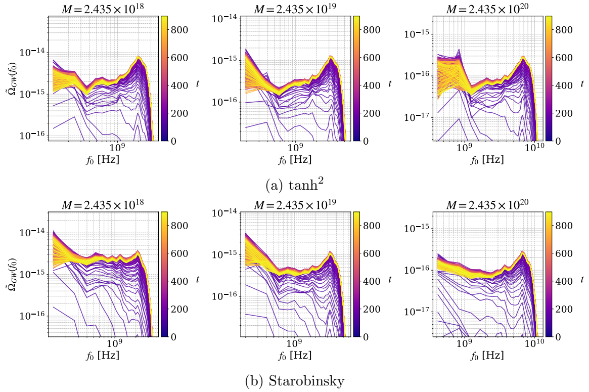
Figura 4.17: Espectro de ondas gravitacionales evaluado para distintos anchos de la meseta (parametrizados por M ) conservando la masa efectiva m constante. Mayores valores de M trasladan la potencia hacia modos ultravioletas y deprimen la señal estocástica total.
